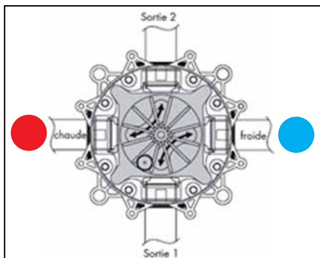
Situation en cas de montage correcte.
