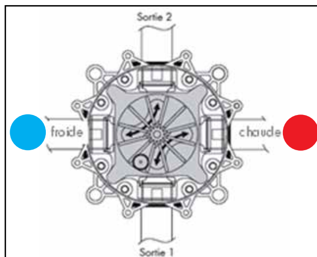
Situation en cas d'inversion entre raccord eau froide et eau chaude.
