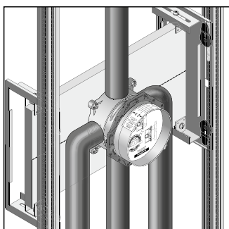
Montage sur système de support
