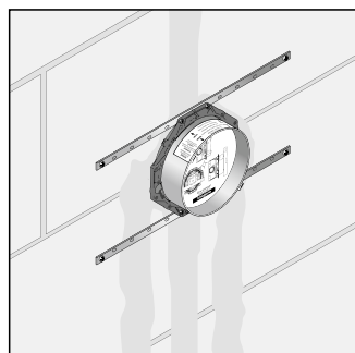
Installation avec kit de rails de montage
