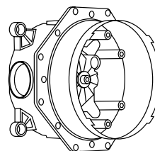
iBox® universal Corps d'encastrement iBox universal # 01800180 Rallonge 25 mm en cas d'encastrement trop profond : # 13595000 Rosace 22 mm en cas d'encastrement trop faible : # 13593000 pour ShowerSelect d'un diamètre de 155 mm x 155 mm # 13597000 pour ShowerSelect d'un diamètre de 150 mm
