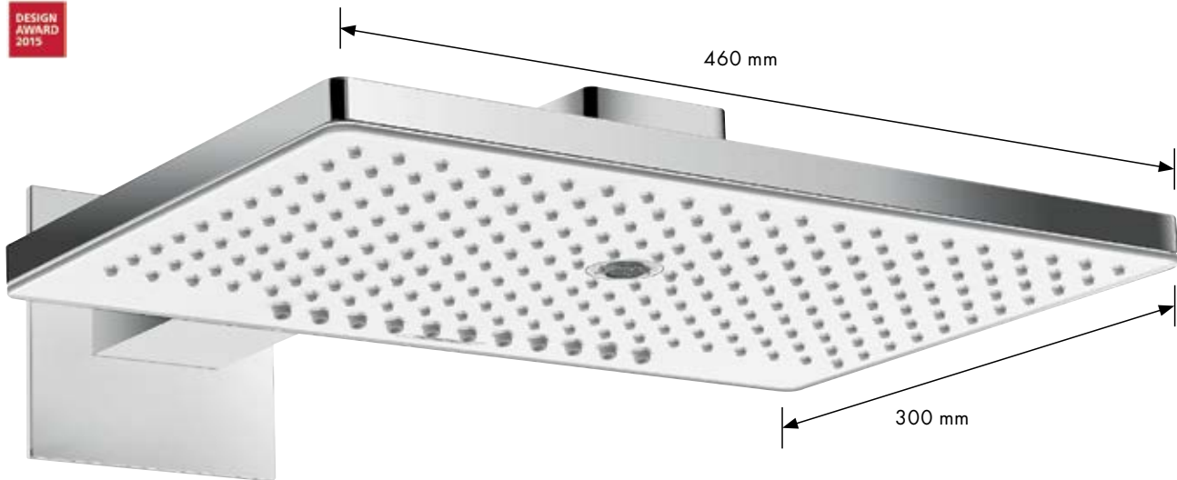
Rainmaker® Select 460 3jet Douche de tête
