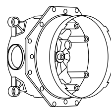
iBox® universal Corps d'encastrement iBox universal # 01800180 Rallonge 25 mm en cas d'encastrement trop profond : # 13595000 Rosace 22 mm en cas d'encastrement trop faible : # 13596000 pour rosaces d'un diamètre de 170 mm # 13597000 pour rosaces d'un diamètre de 150 mm # 97407000 pour rosaces d'un diamètre de 172 mm # 15597000 pour PuraVida
