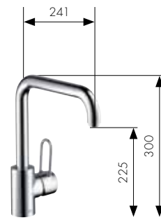
Mitigeur Cuisine avec bec pivotant Réf. 14850000 chauffe-eau instantané Réf. 14852000 robinet d'arrêt (pas d'illustration) Réf. 14855000
