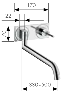
Mitigeur Cuisine Version encastrée Réf. 38815, -000, -800 Corps d'encastrement (pas d'illustration) Réf. 13622180
