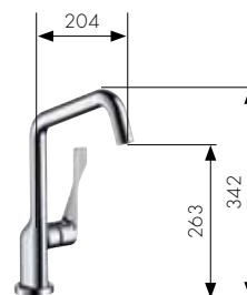
Mitigeur Cuisine avec bec pivotant Réf. 39850, -000, -800 chauffe-eau instantané Réf. 39852, -000, -800
