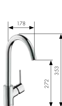
Mittigeur Cuisine avec bec pivotant Réf. 14870, -000, -800 chauffe-eau instantané Réf. 14873000
