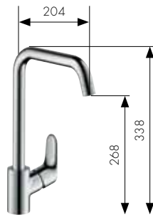
Mitigeur Cuisine avec bec pivotant Réf. 31820, -000, -800 chauffe-eau instantané Réf. 31822, -000, -800
