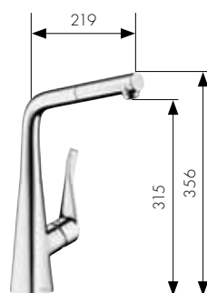
Mittigeur Cuisine avec bec extractible Réf. 14821, -000, -800
