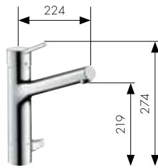
Mitigeur Cuisine robinet d'arrêt Réf. 32855000
