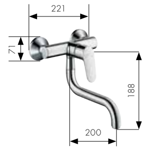
Mitigeur Cuisine pour montage mural Réf. 31825000
