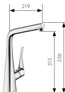
Mittigeur Cuisine avec bec pivotant Réf. 14822, -000, -800 pour montage devant une fenêtre Réf. 14823000
