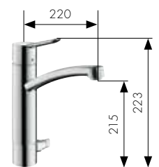
Mitigeur Cuisine robinet d'arrêt Réf. 31783000
