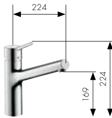
Mitigeur Cuisine Réf. 32851, -000, -800 Débit limité : 5l/min Réf. 32852000
