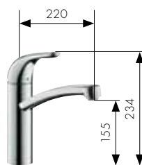
Mitigeur Cuisine Réf. 31780000 chauffe-eau instantané Réf. 31784000
