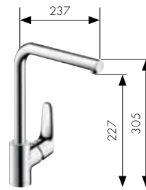
Mitigeur Cuisine avec bec pivotant (bec en L) Réf. 31817, -000, -800
