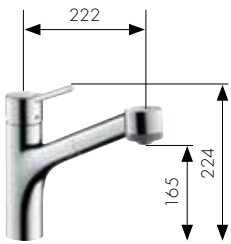
Mitigeur Cuisine avec douchette extractible Réf. 32841, -000, -800 Débit limité : 5l/min Réf. 32842000
