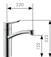
Mitigeur Cuisine Réf. 31786000 chauffe-eau instantané Réf. 31785000
