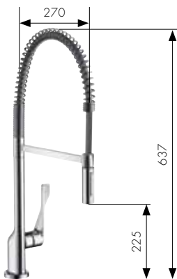
Mitigeur Cuisine Semi-Pro Réf. 39840, -000, -800
