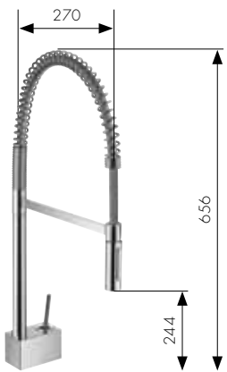
Mitigeur Cuisine Semi-Pro Réf. 10820000
