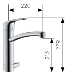
Mitigeur Cuisine robinet d'arrêt Réf. 31803000
