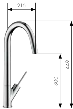
Mitigeur Cuisine avec bec pivotant Réf. 10822, -000, -800
