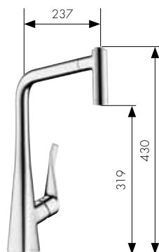
Mittigeur Cuisine avec douchette extractible Réf. 14820, -000, -800
