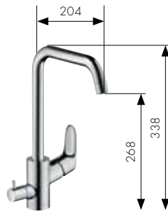
Mitigeur Cuisine avec bec pivotant robinet d'arrêt Réf. 31823000
