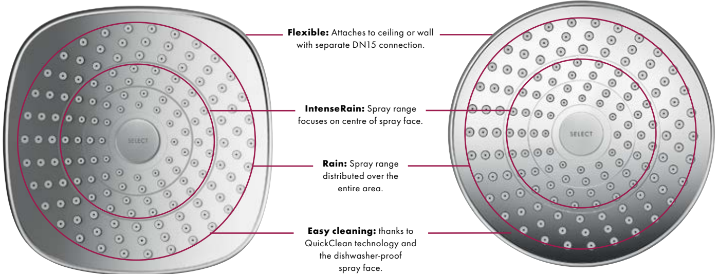
Croma® Select E 180 2jet
