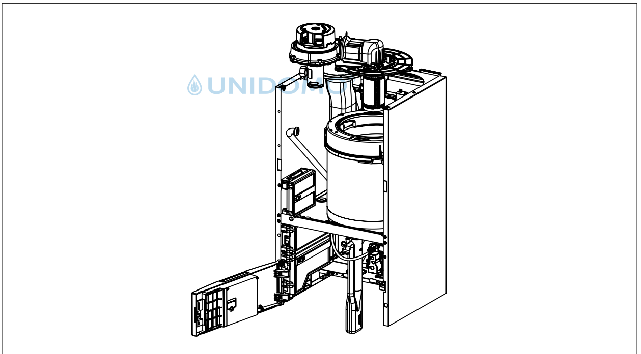
Abb. 5.9 Brennkammerdeckel abheben
