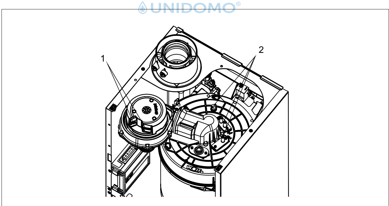
Abb. 5.7 Anschlusskabel Brennkammerdeckel lösen
