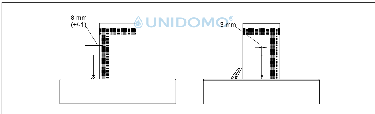
Abb. 6.4 Abstände Ionisationselektrode
