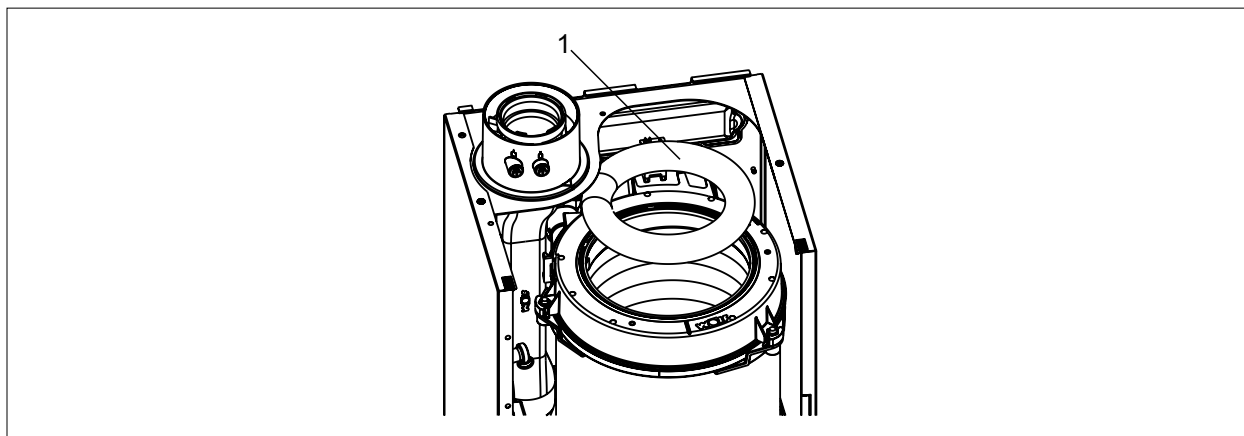
Abb. 6.7 Isolerring herausnehmen
