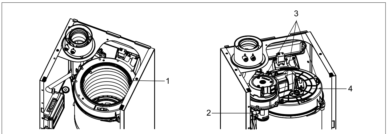
Abb. 6.11 Brennkammerdeckel montieren
