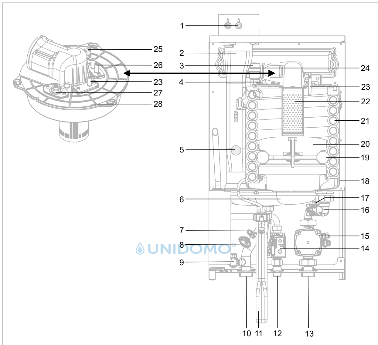
Abb. 4.1 Aufbauschema Gasbrennwerttherme
