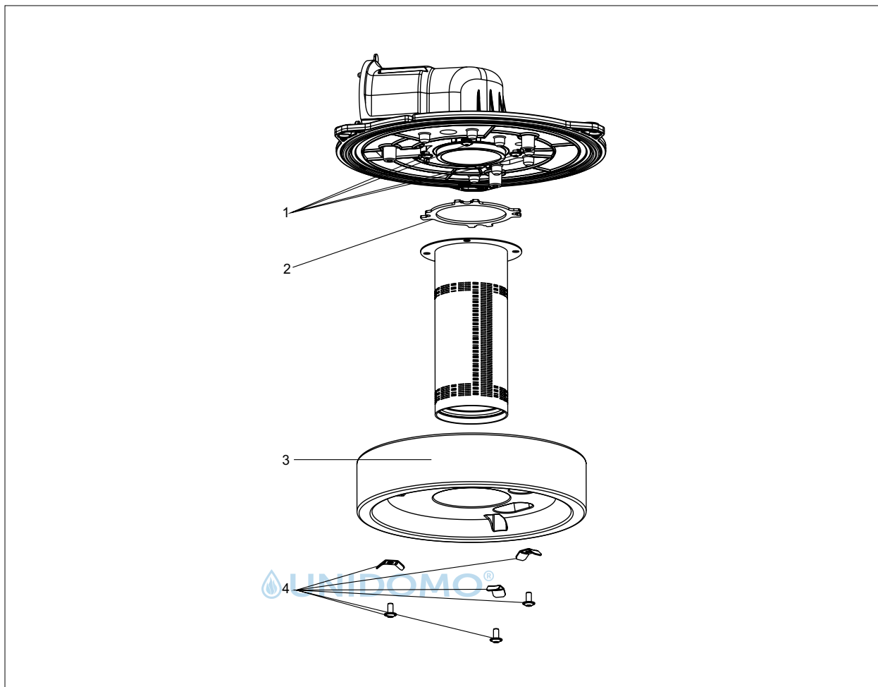
Abb. 6.2 Brenner zerlegen
