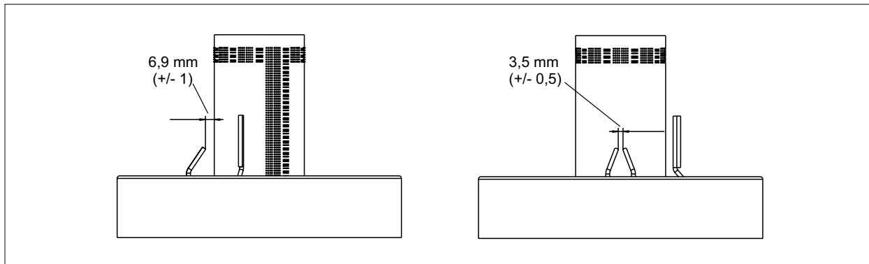
Abb. 6.5 Abstände Zündelektrode
