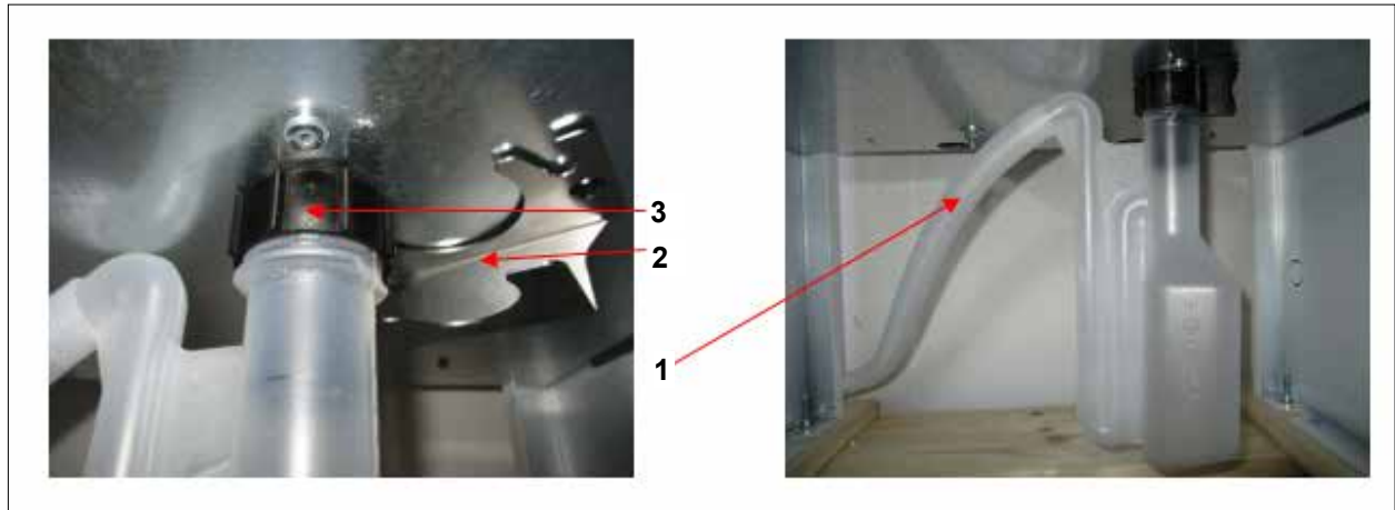
Abb. 5.16 Siphon demontieren
