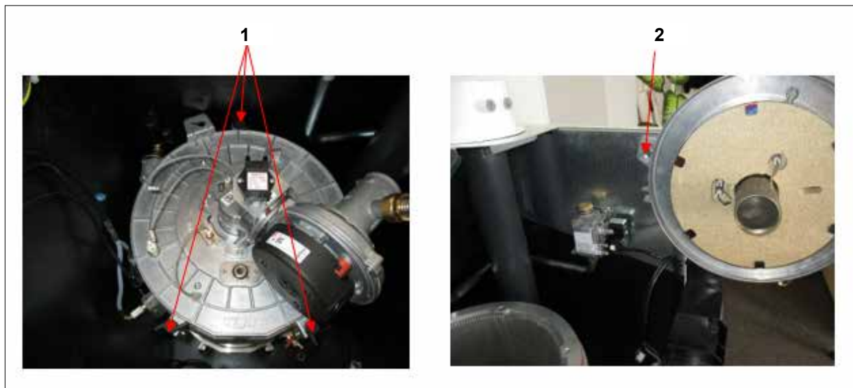
Abb. 5.11 Brennerdeckel Wartungsposition
