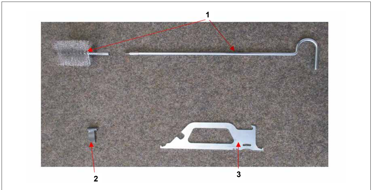
Abb. 5.2 Wartungswerkzeuge von WOLF 1 Reinigungsbürste (2-teilig) 3 Wartungswerkzeug 2 Reinigungshaken
