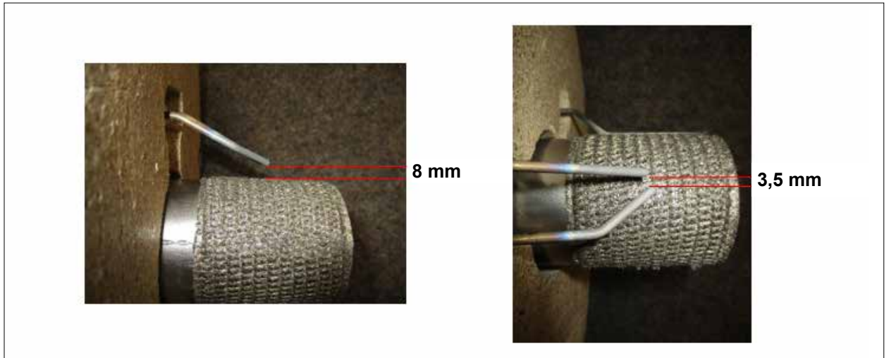
Abb. 5.14 Abstände Zündelektrode
