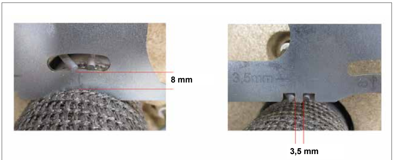
Abb. 5.15 Abstände Zündelektrode mit Wartungswerkzeug
