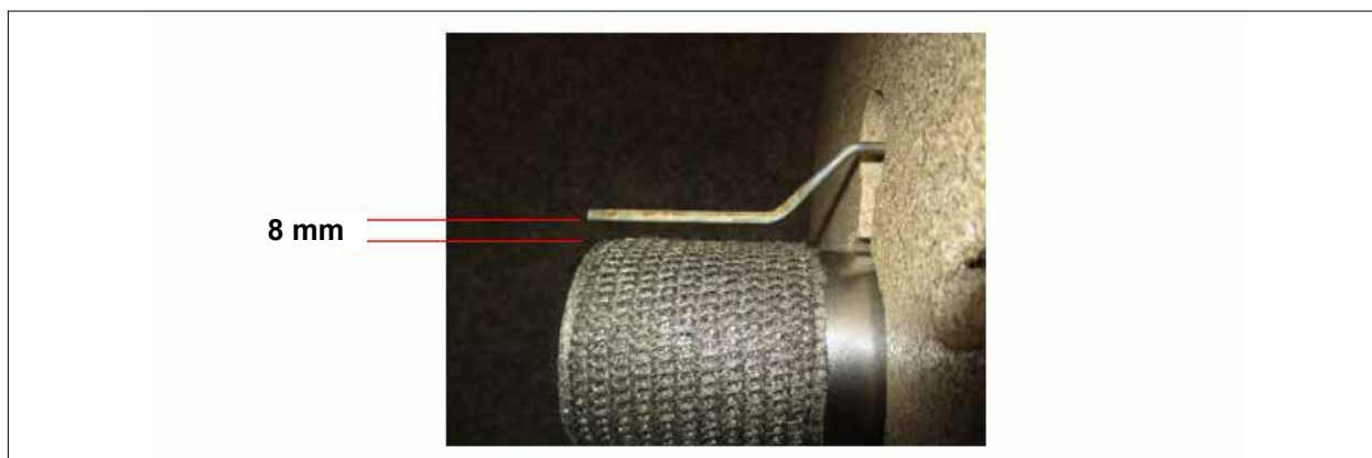
Abb. 5.12 Abstand Ionisationselektrode
