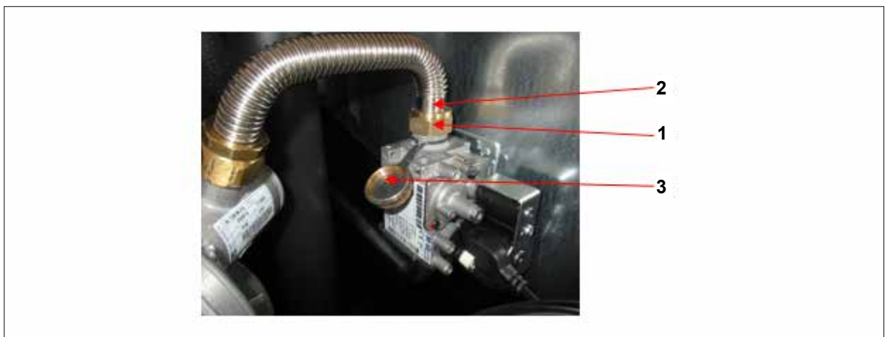
Abb. 5.24 Gaswellrohr anschliessen
