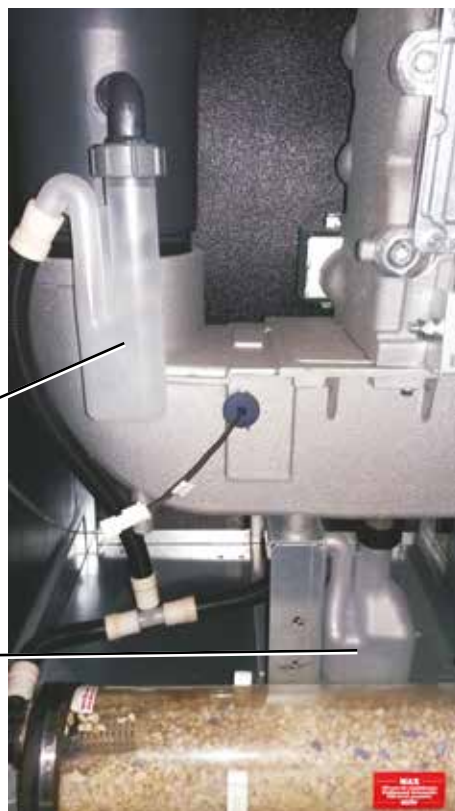
Siphon Kondensat-falle
