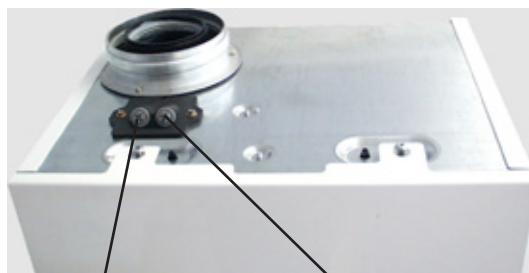
Messöffnung „Abgas“
