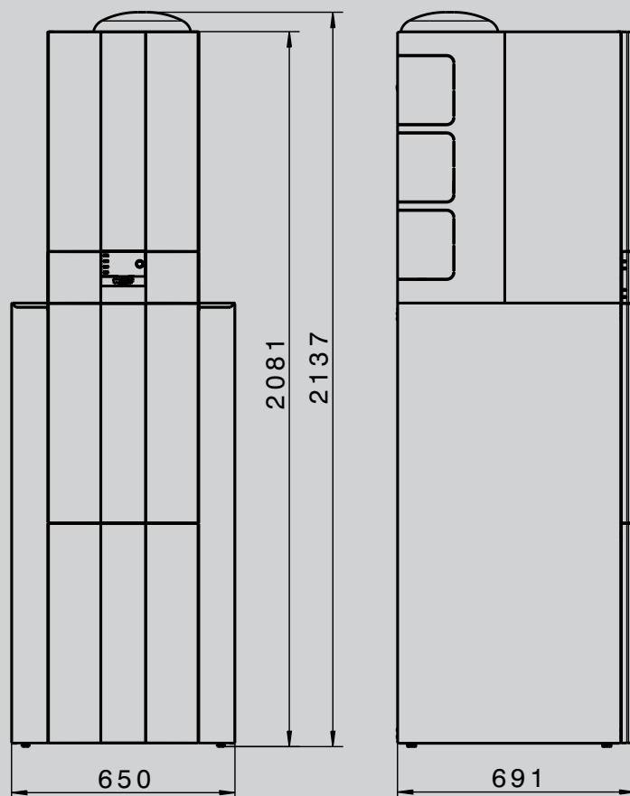
Vorderansicht
