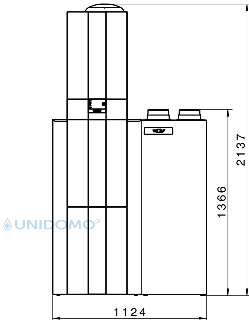
Vorderansicht
