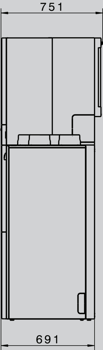
Seitenansicht
