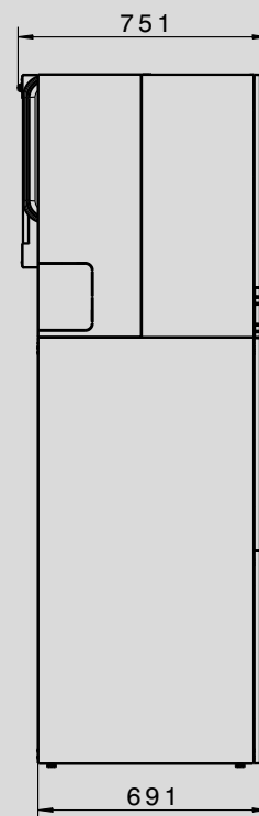
Seitenansicht
