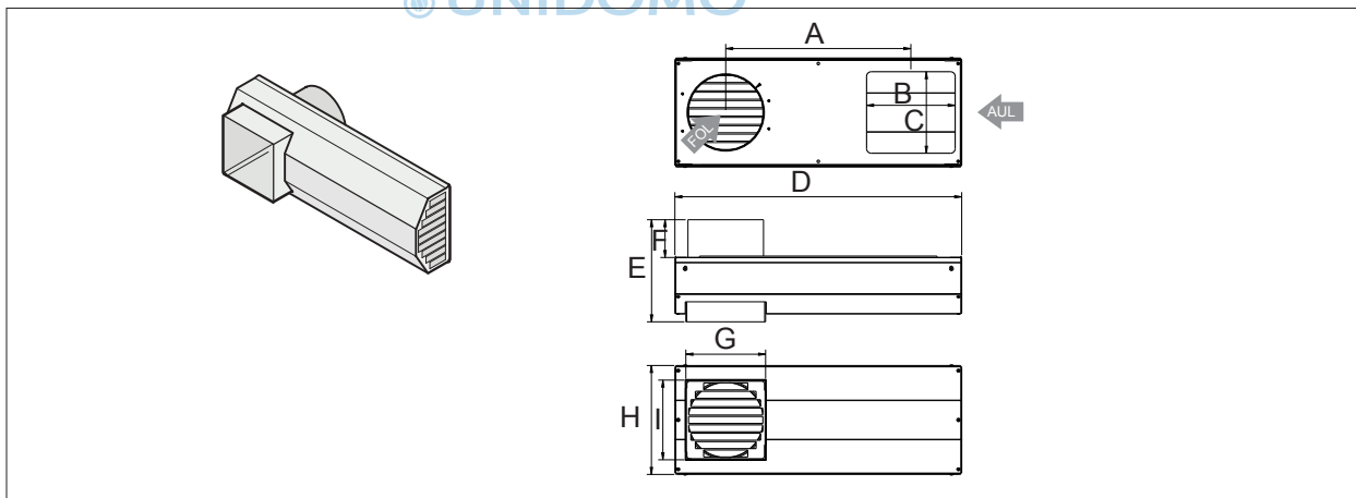
Abb. 9.4 Doppelgitter Edelstahl
