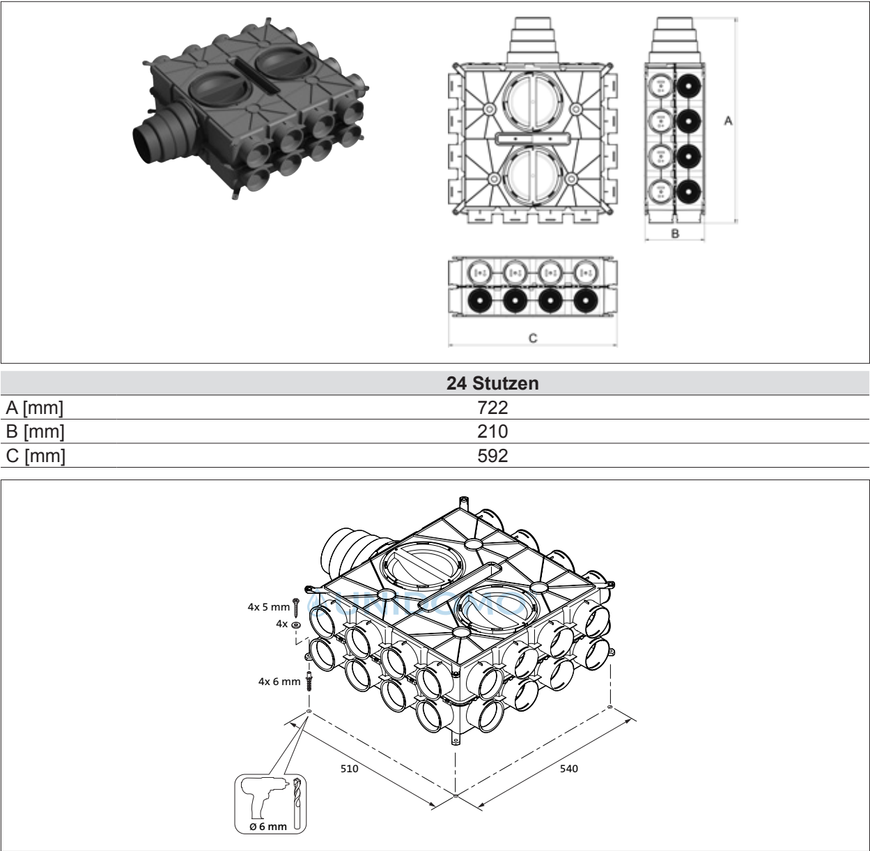
Abb. 4.1 Abstände Bohrlöcher
