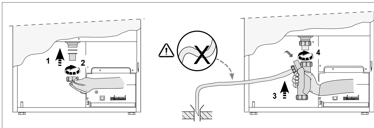
Abb. 11.22 Siphon montieren
