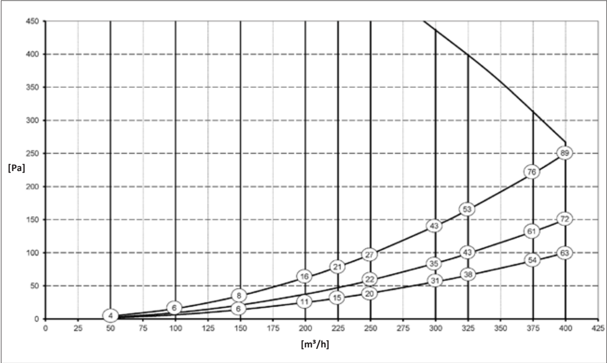
Abb. 11.7 Ventilator Kennlinie CWL-2-400 [Pa] Luftwiderstand im Kanalsystem [m³/h] Volumenstrom Die in den Kreisen gezeigten Zahlen stellen jeweils die Leistung (in Watt) je Ventilator dar.
