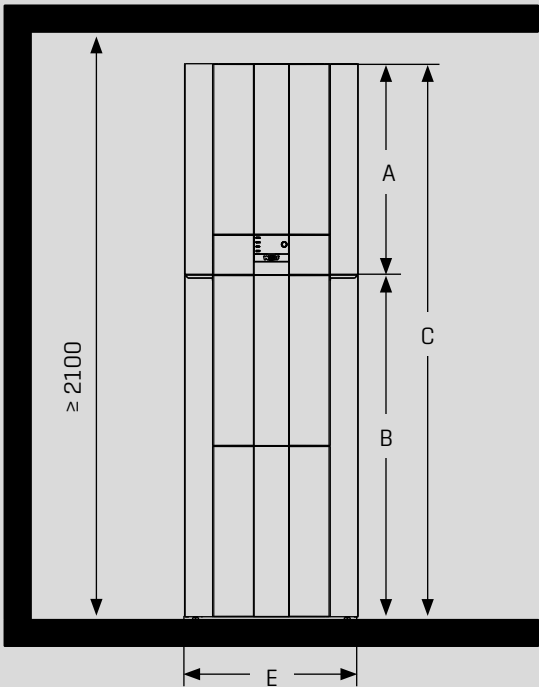
Vorderansicht CHC-Split /200-35
