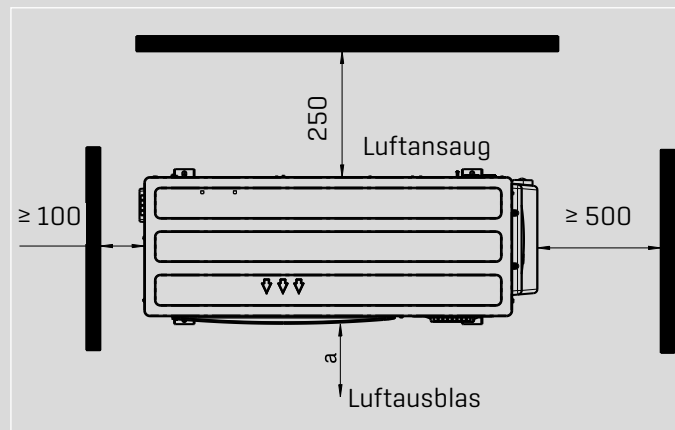
Abb. Draufsicht Außenmodul BWL-1S(B)-10/14/16
