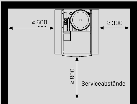
Draufsicht CHC-Split /200
