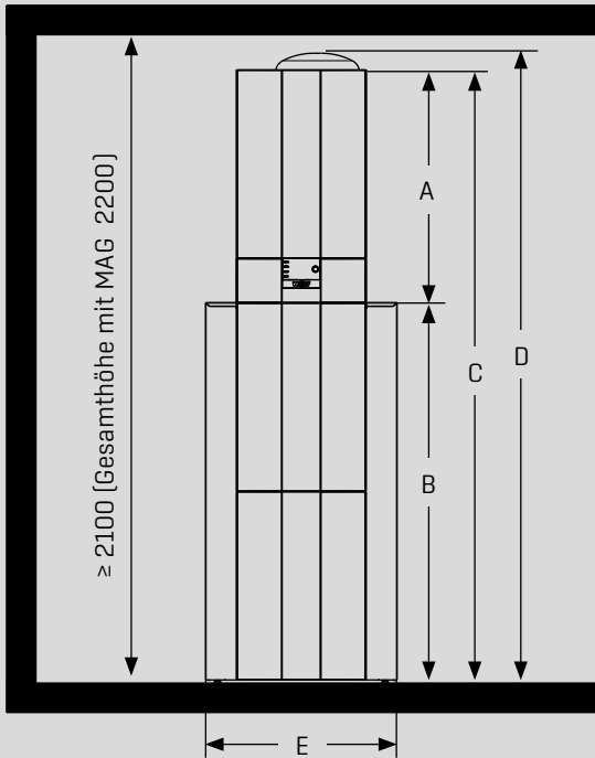
Vorderansicht CHC-Split /200
