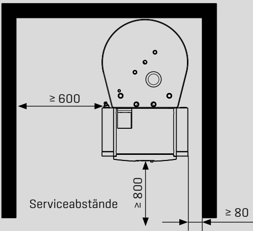
Draufsicht CHC-Split /300
