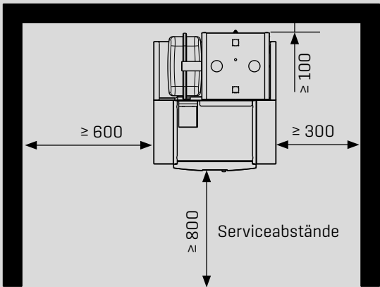
Draufsicht CHC-Split /200-35
