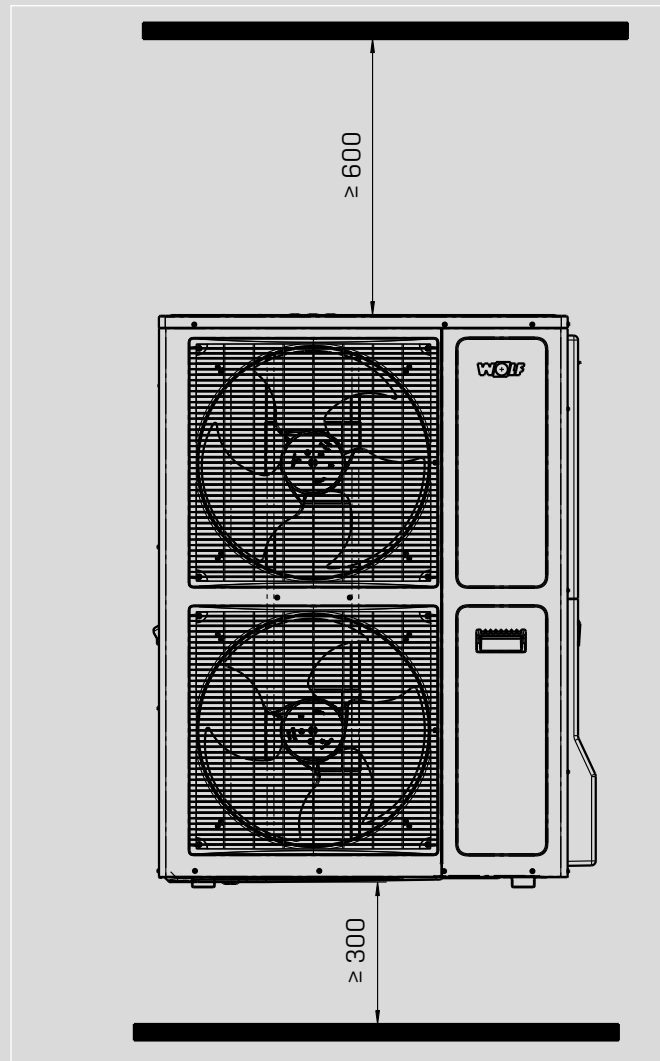
Abb. Frontansicht Außenmodul BWL-1S(B)-10/14/16
