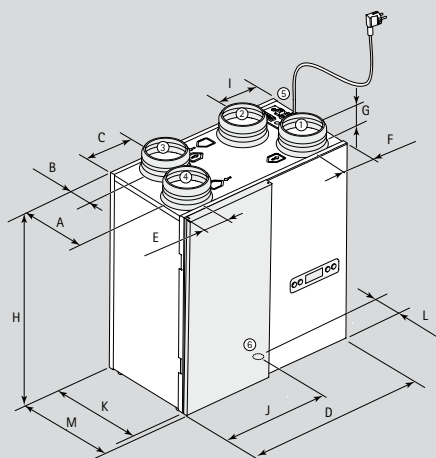
Anschluss 4/0 L
