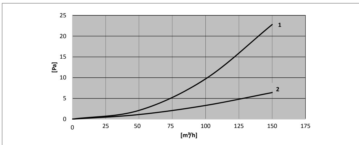
Abb. 9.5 Druckverlust DN 125
