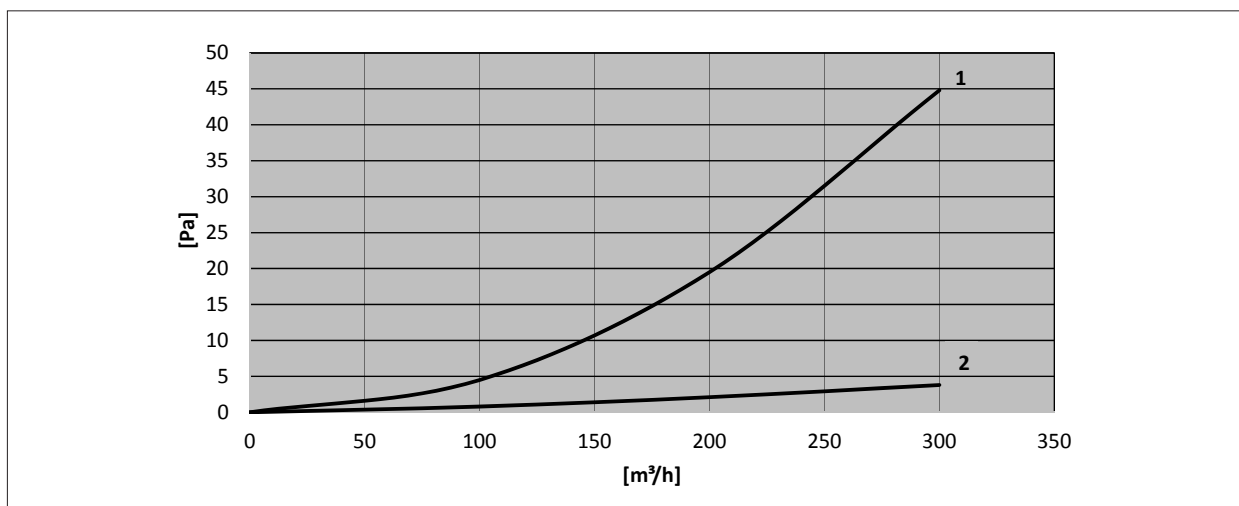
Abb. 9.6 Druckverlust DN 160
