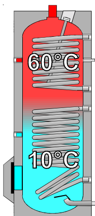
Optimale Temperaturschichtung
