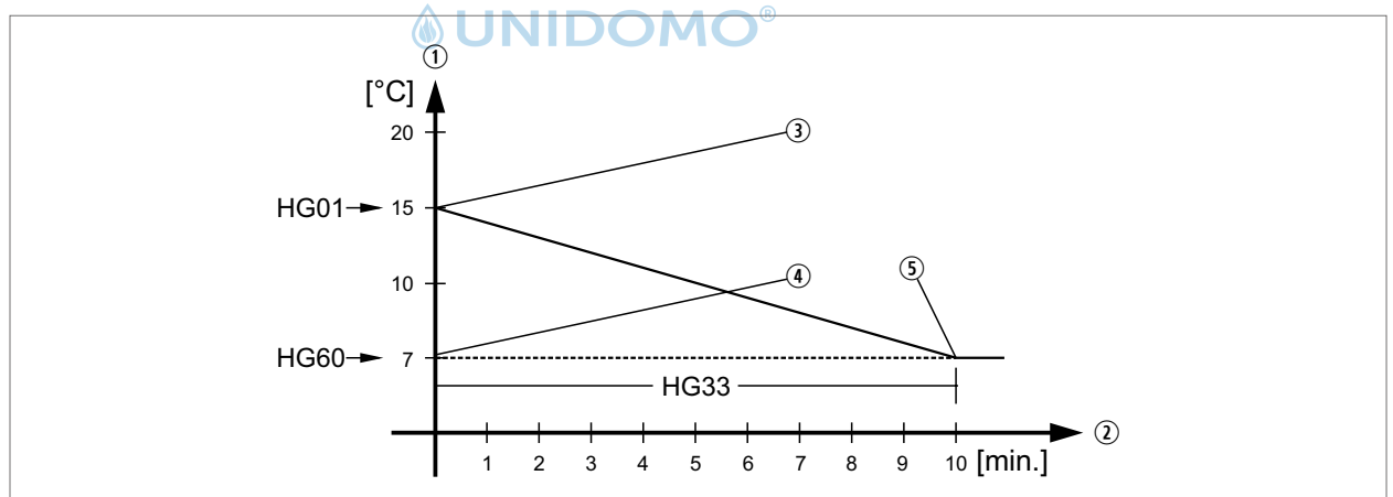
Abb. 7.1 Brennerhysterese
