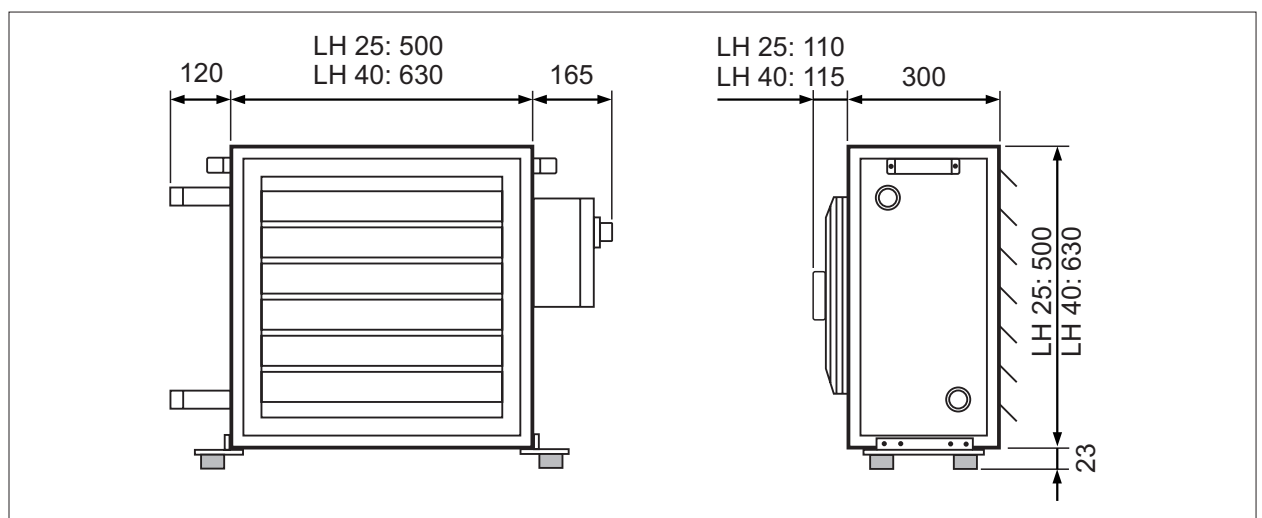
Abb. 11.1 Abmessungen
