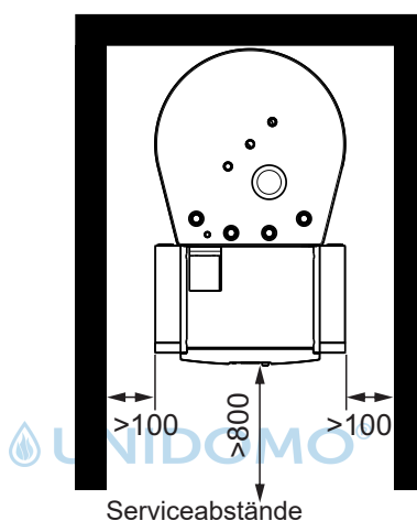
Draufsicht CHC-Monoblock /300
