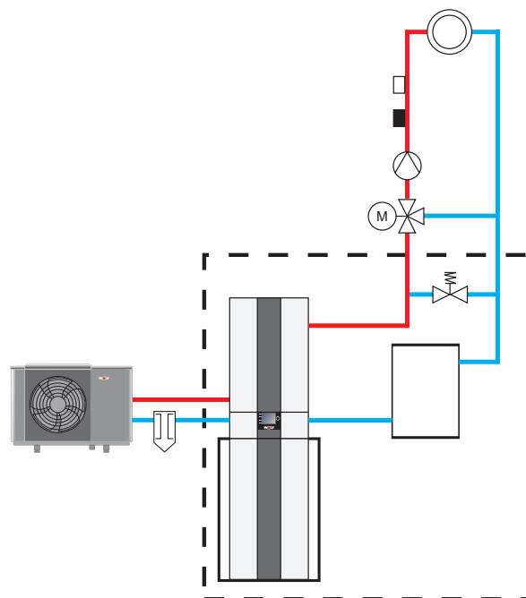
Wärmepumpencenter mit Reihenspeicher und Überströmventil (im System integriert) und Mischerkreis
