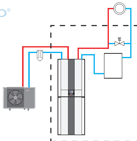
Wärmepumpencenter mit Reihenspeicher und Überströmventil (im System integriert) und Mischerkreis
