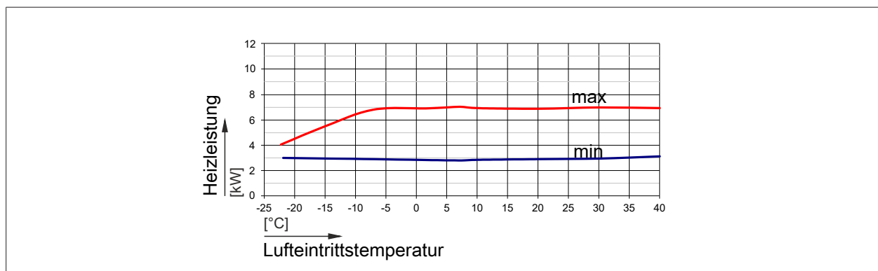
Abb. 7: Heizleistung bei einem Vorlauf von 35 °C
