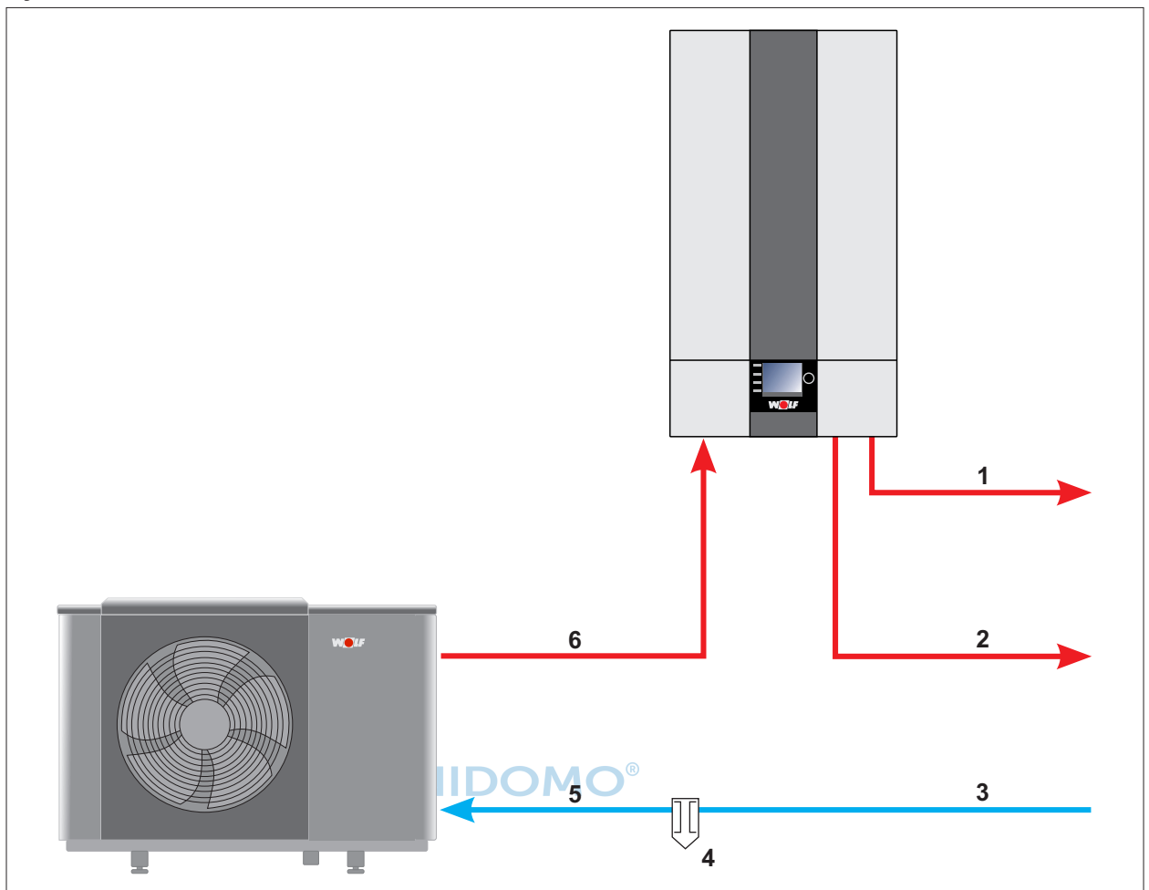
Abb. 5.15 Hydraulisches Schema
