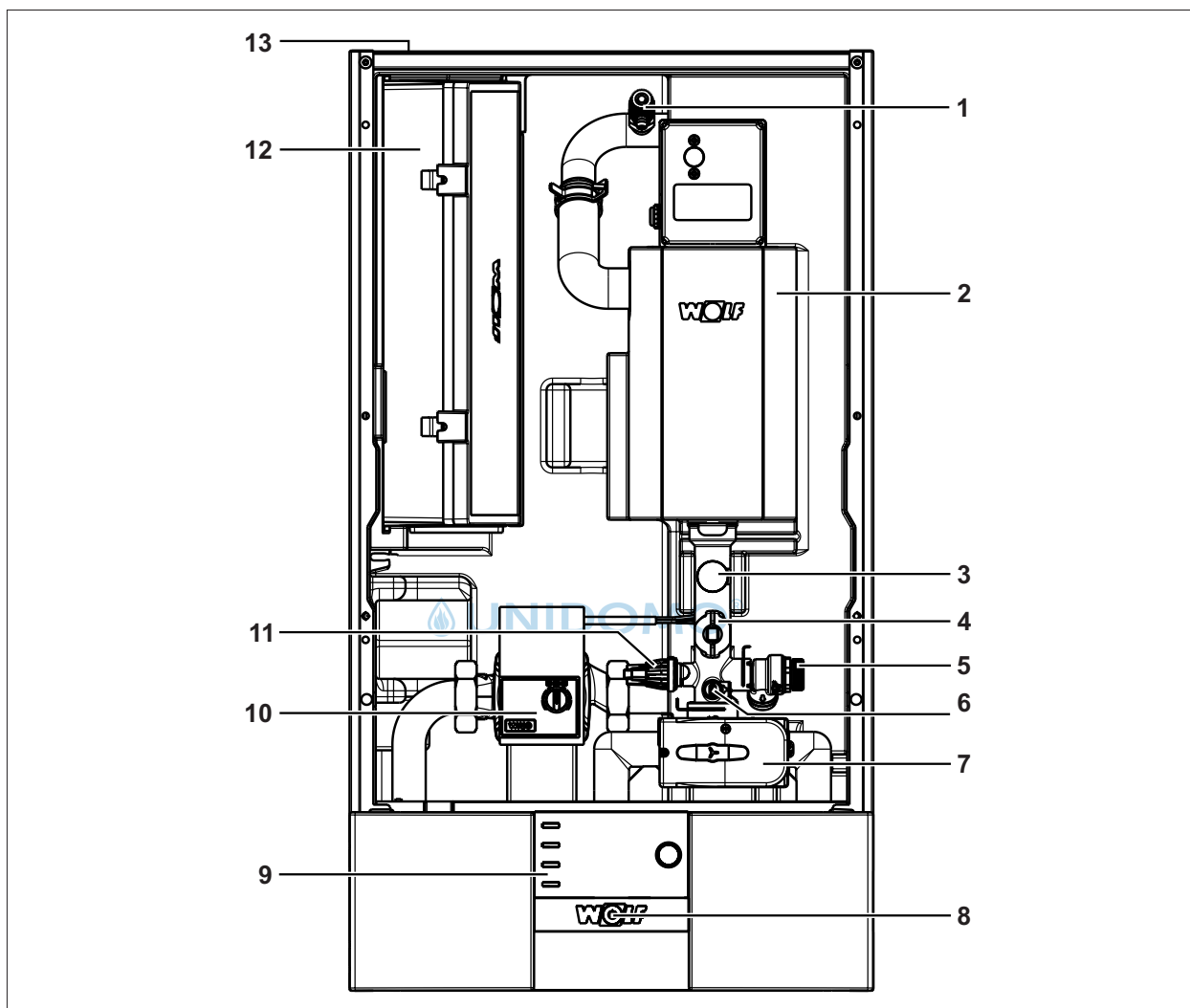
Abb. 3.1 Bauteile Inneneinheit
