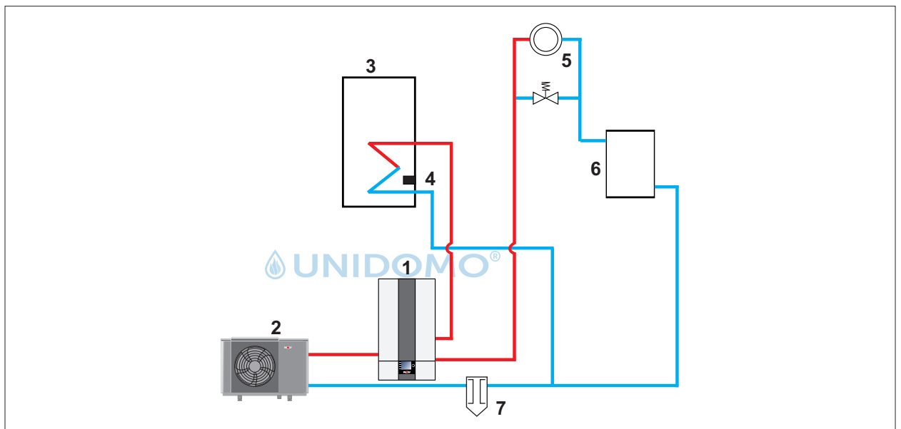
Abb. 17.3 Anlagenkonfiguration 01, Beispiel 1
