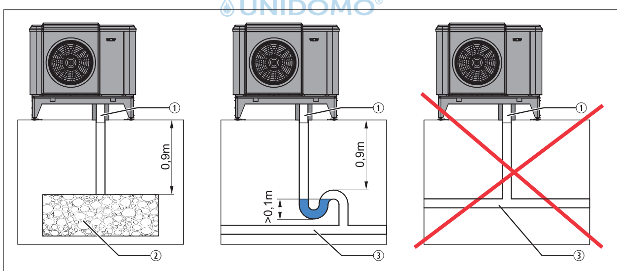
Abb. 4.9 Kondensatablauf
