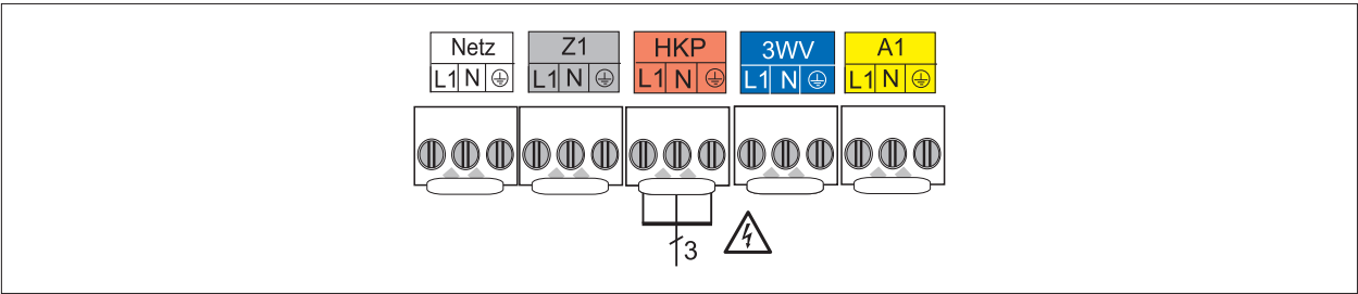
Abb. 5.32 Anschluss Heizkreispumpe
