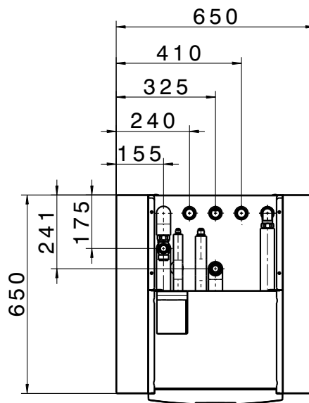
Draufsicht
