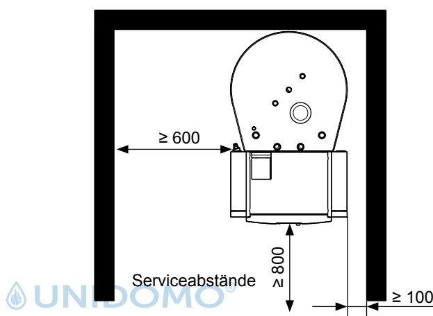
Draufsicht CHC-Split /300
