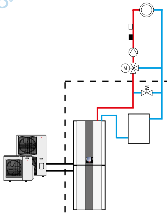
Wärmepumpencenter mit Reihenspeicher und Überströmventil (im System integriert) und Mischerkreis
