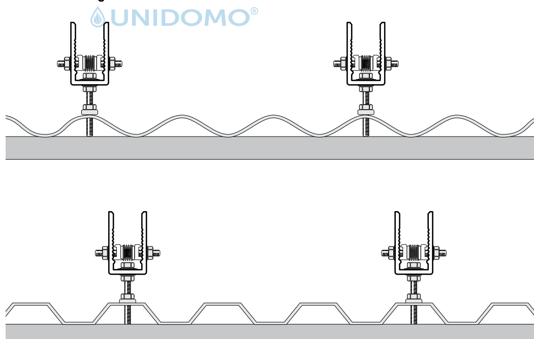
Dachhaken montiert
