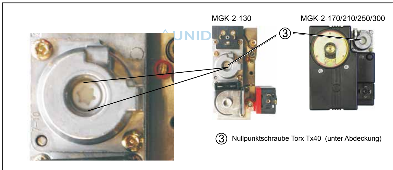
Bild: Gaskombiventil
