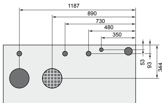
MGK-2-170/210/250/300
