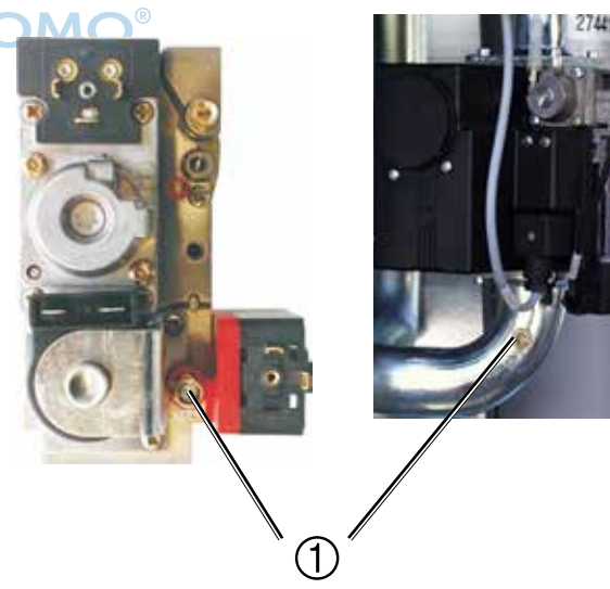
Bild: Messnippel zum Überprüfen des Gasanschlussdrucks
