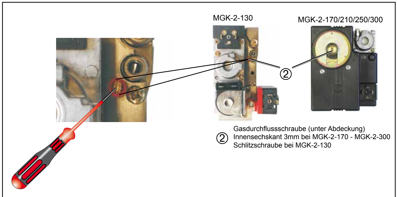
Bild: Gaskombiventil
