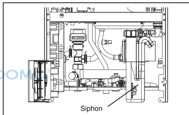
Bild: Siphon
