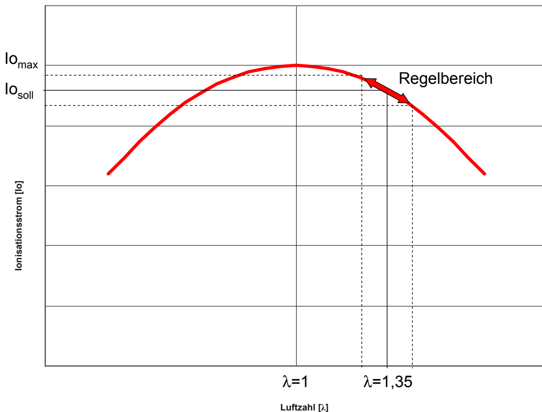
Bild: Diagramm Ionisationsstromregelung
