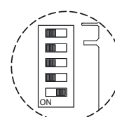
Richtige Einstellung Mikroschalter CWL-180 Excellent mit Erweiterungssatz
