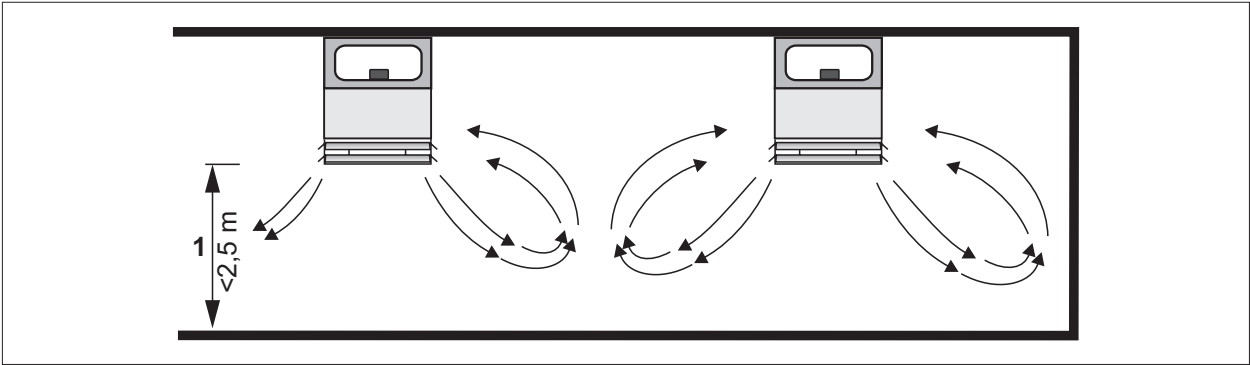
Abb. 4.7 Wurfweiteckengerät, Luftrichtung vertikal mit Vierseitenausblas
