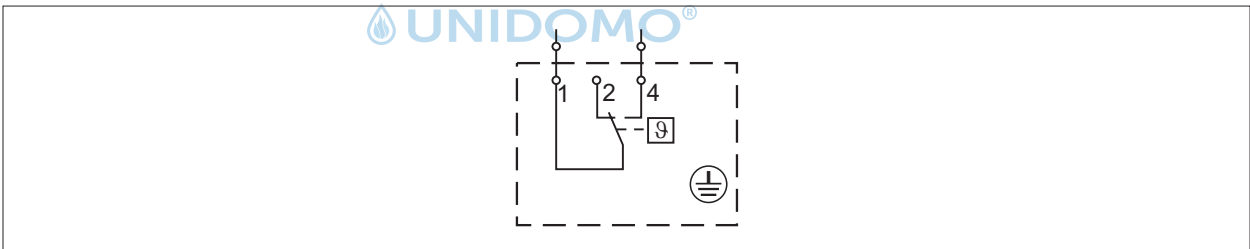
Abb. 7.22 Schaltplan Frostschutzthermostat
