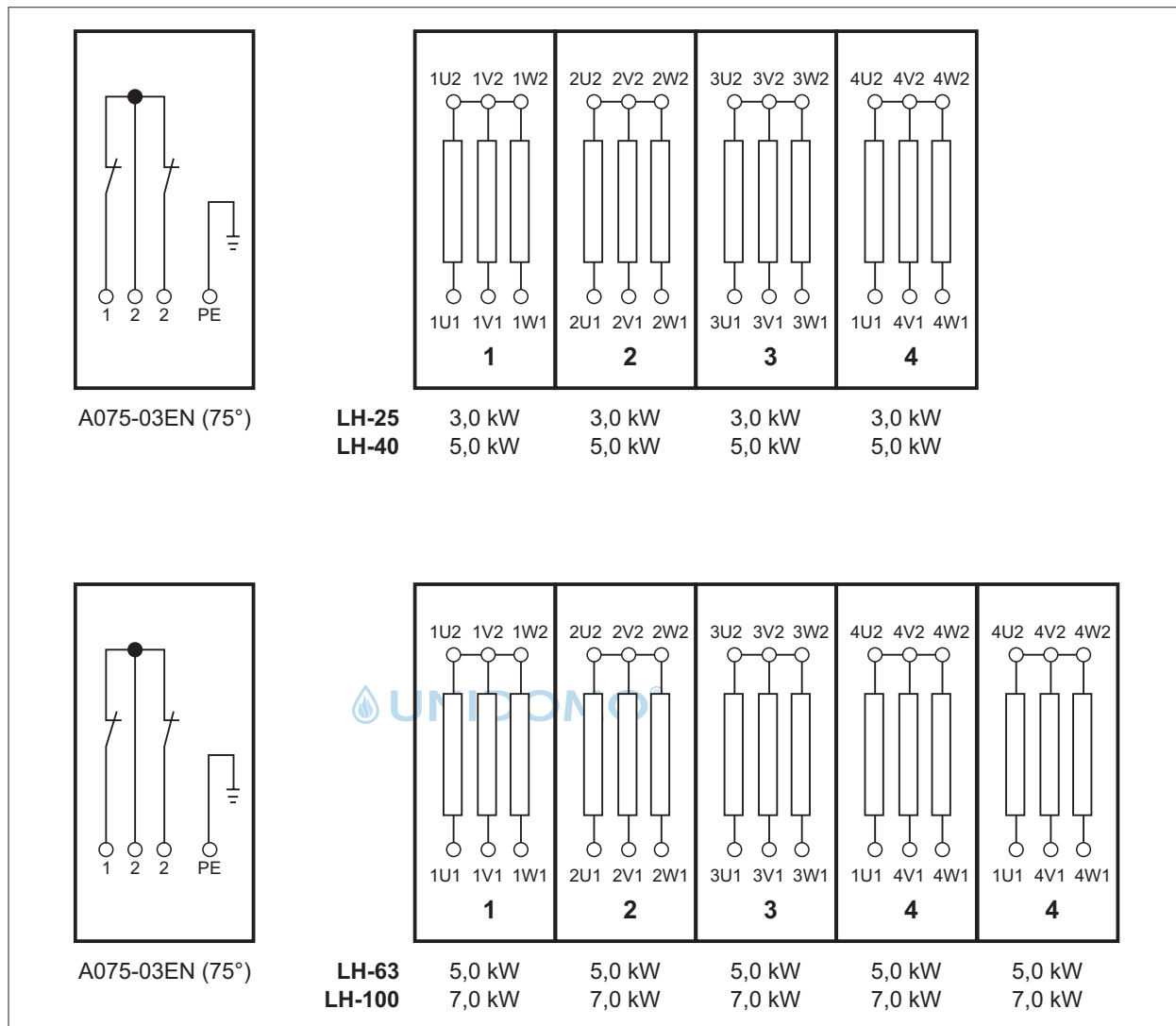
Abb. 5.12 Schaltplan Elektroheizregister
