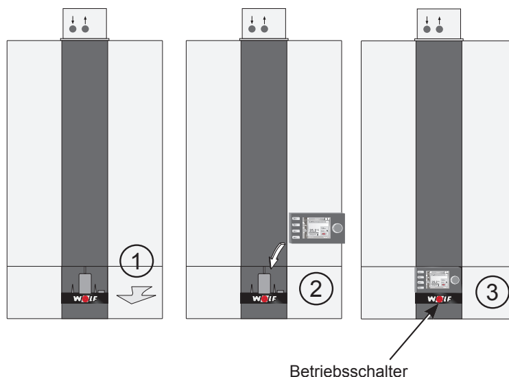
Abb. 4.1 Bedienmodul BM-2 einsetzen
