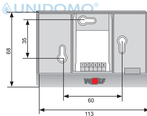
Abb. 4.6 Wandsockel BM-2 mit Schrauben und Dübeln an Wand montieren
