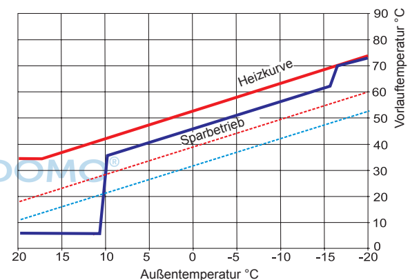
Temperaturanpassung +4 Heizkurve Heizkreis wird angehoben
