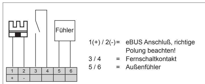
Abb. 4.8 Klemmenblockbelegung Wandsockel
