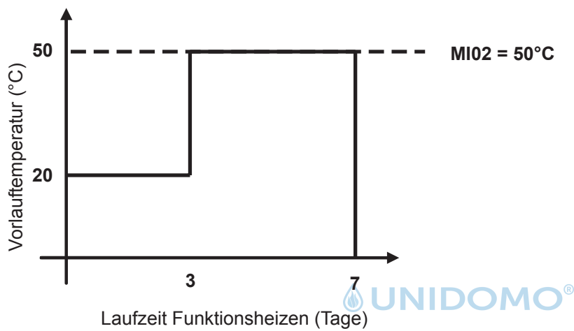
Abb. 26.2 Zeitlicher Verlauf der Vorlauftemperatur Mischerkreis während Funktionsheizen.
