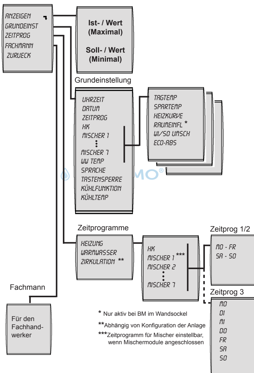
Abb. 5.1 Menüstruktur Bedienmodul BM
