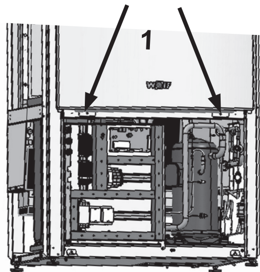
Schrauben montieren
