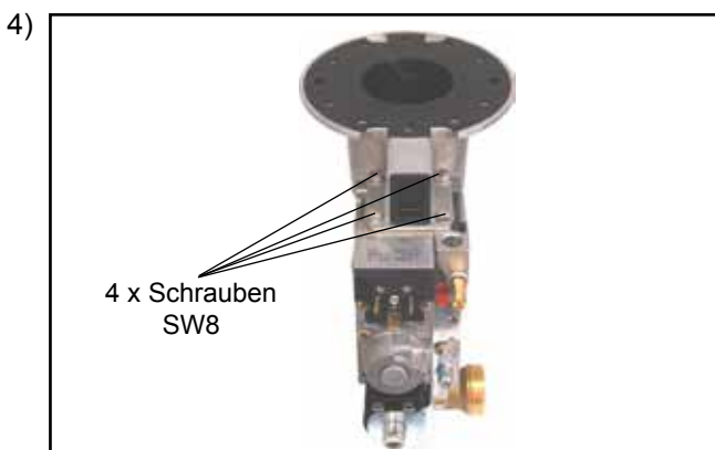
Gaskombiventil von der Mischkammer für Gas/Luft abschrauben (4 Schrauben SW8).
