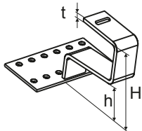
Haken Falz-Ziegel t = 6 oder 8 mm h = 45 mm H = 130 mm
