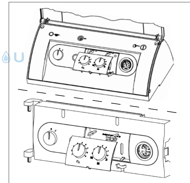
Abb. 4.8 Frontblende herausnehmen
