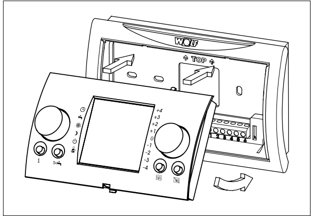
Abb. 4.7 Bedienmodul BM in Wandschalter einsetzen
