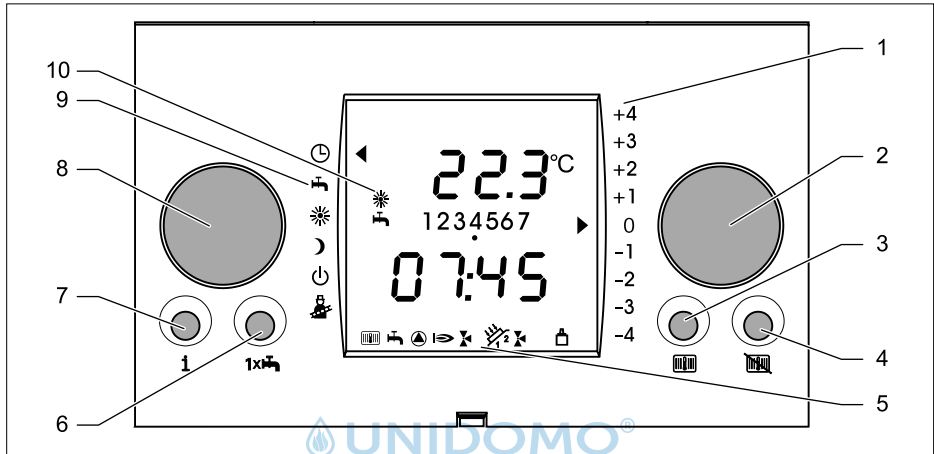
Abb. 5.1 Bedienmodul BM
