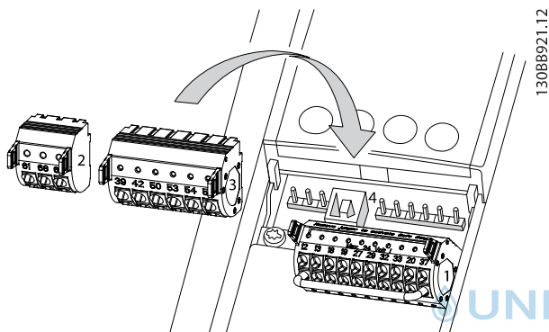
Abbildung 4.8 Anordnung der Steuerklemmen
