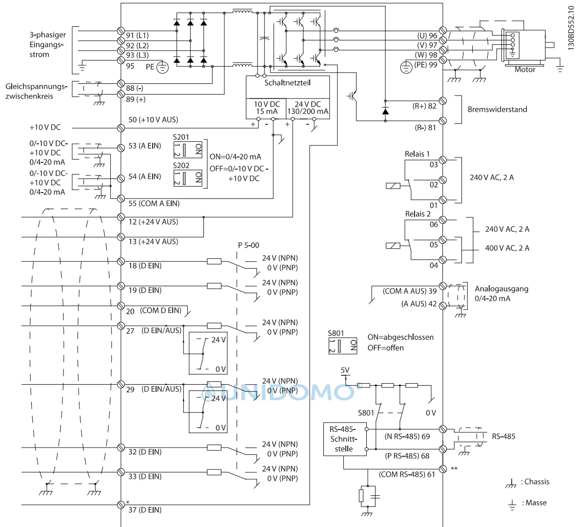
Abbildung 4.2 Anschlussdiagramm des Grundgeräts
