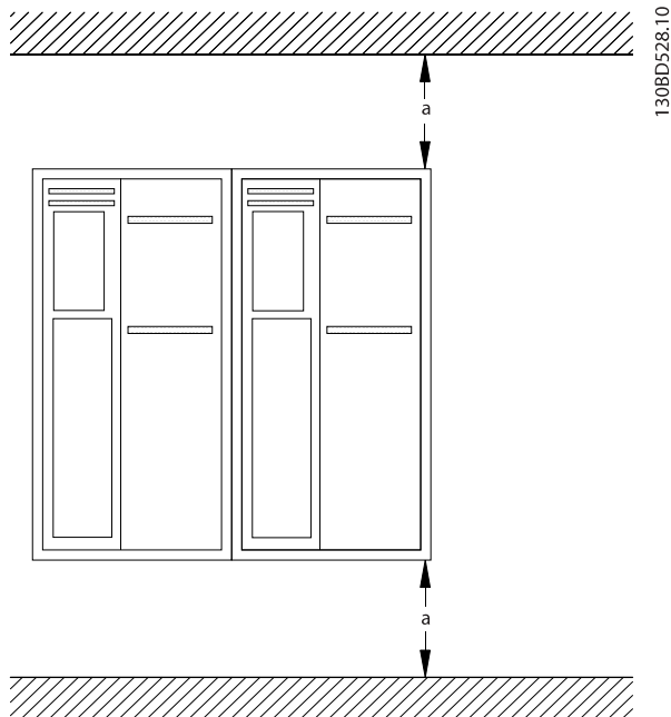
Abbildung 3.3 Ordnungsgemäße Montage mit Rückwand
