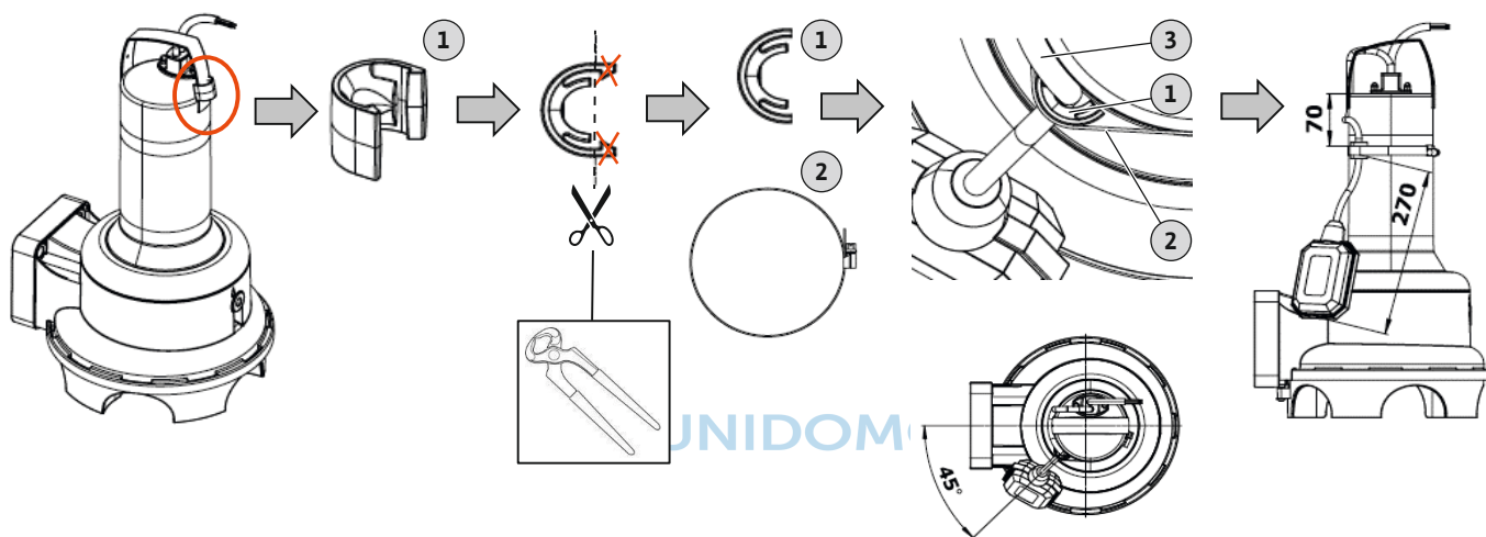
Fig. 15: Rexa UNI: Lunghezza cavo interruttore a galleggiante
