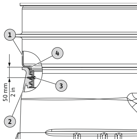
Fig. 12: Schachtverlängerung montieren
