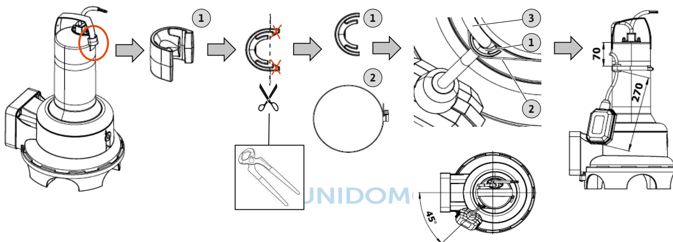
Fig. 15: Rexa UNI : longueur du câble de l'interrupteur à flotteur
