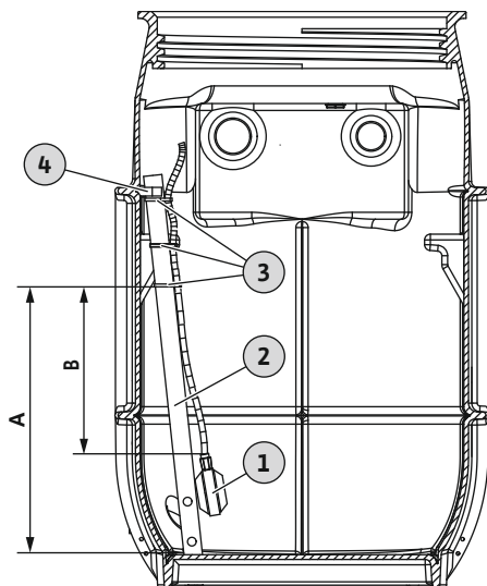
Fig. 16: Installation Schwimmerschalter
