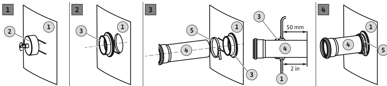
Fig. 8: Raccordement de l'arrivée
