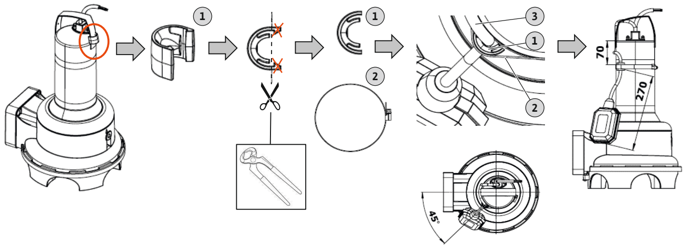
Fig. 15: Rexa UNI: Kabellänge Schwimmerschalter
