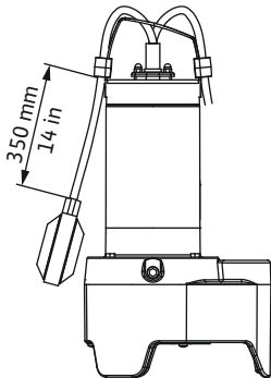
Fig. 14: Rexa MINI3: Kabellänge Schwimmerschalter
