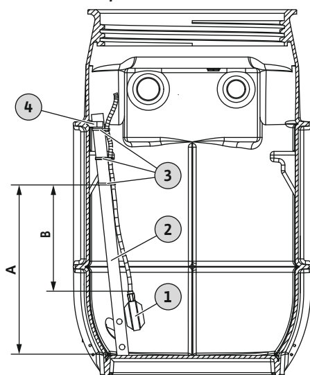
Fig. 16: Montage de l'interrupteur à flotteur
