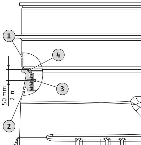
Fig. 12: Montage de l'extension de cuve
