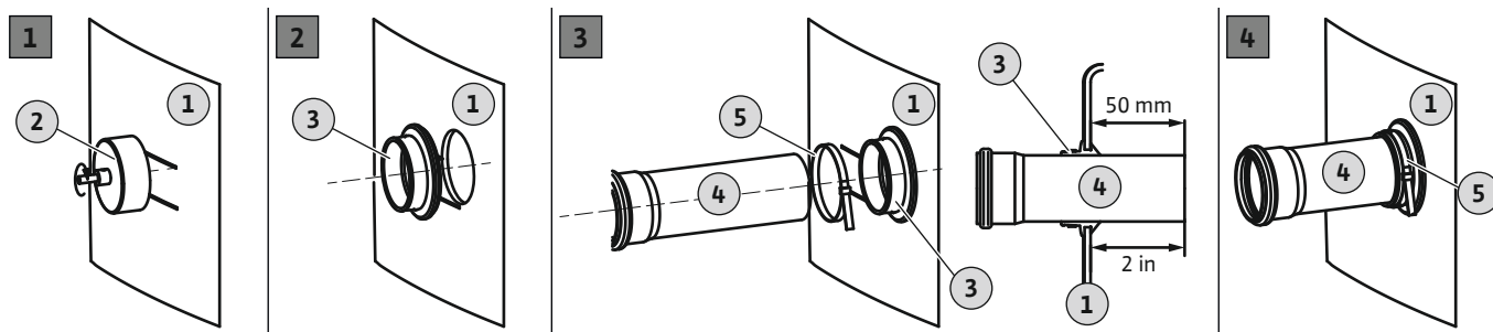
Fig. 8: Zulauf anschließen
