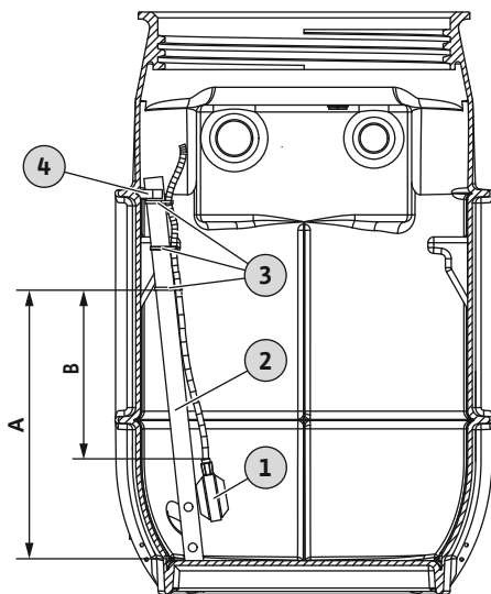
Fig. 16: Installazione interruttore a galleggiante
