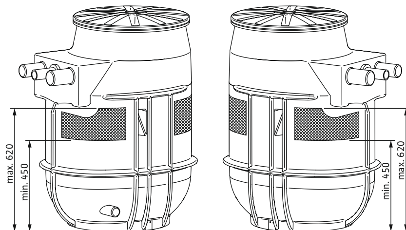
Fig. 7: Surfaces d'arrivée
