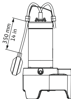
Fig. 14: Rexa MINI3: Lunghezza cavo interruttore a galleggiante
