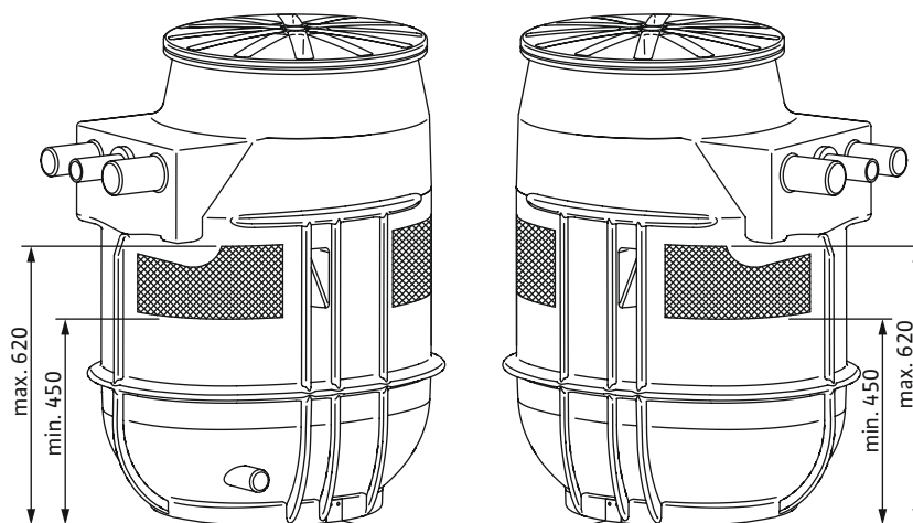
Fig. 7: Zulaufflächen
