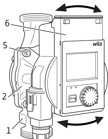
Fig. 3: Motorkopf drehen
