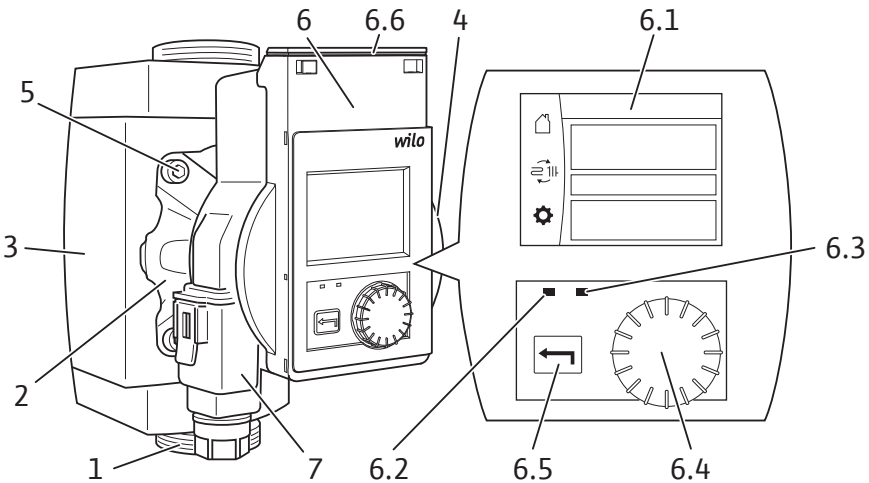
Fig. 1: Übersicht
