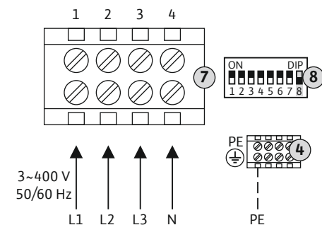
Fig. 7: Netzanschluss 3~400 V ohne Hauptschalter
