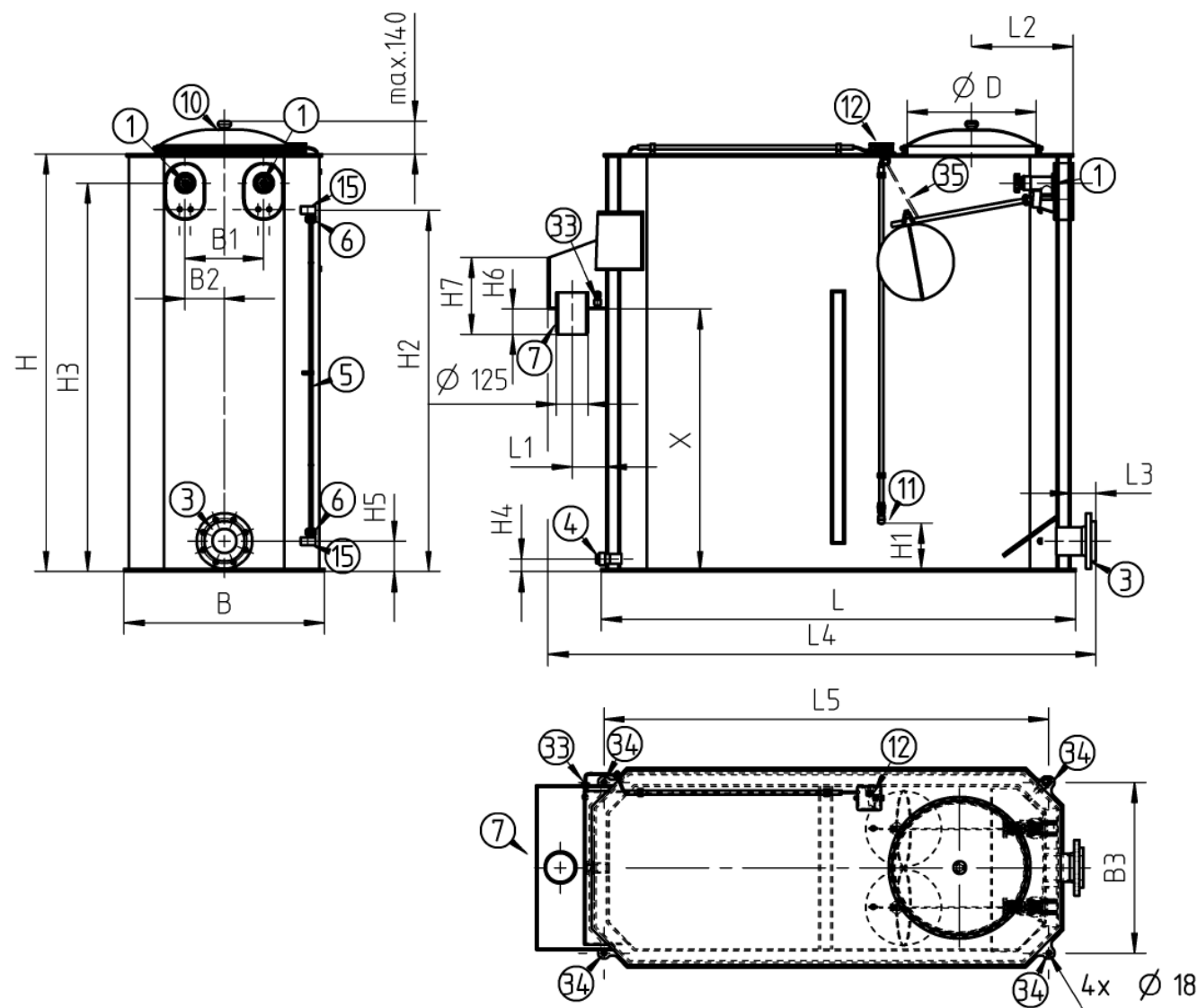
W-VORBEHÄLTER 1080L-VT-ECK-2xG2-ACS
