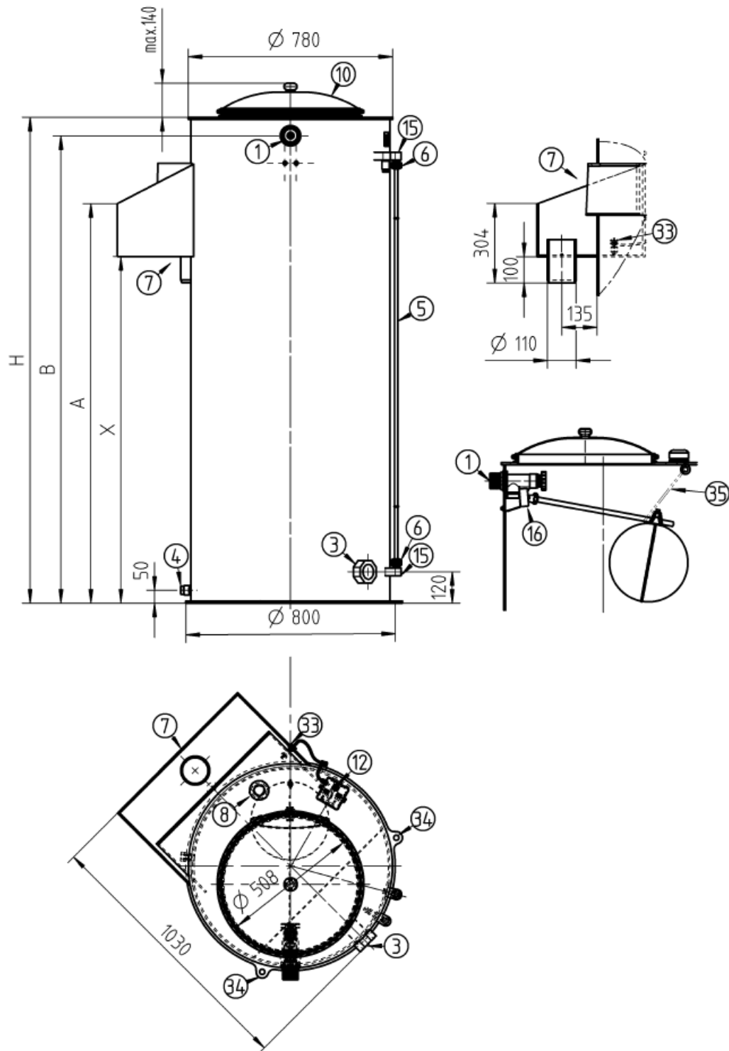
W-VORBEHÄLTER 540L-VT-RD-G2-ACS
