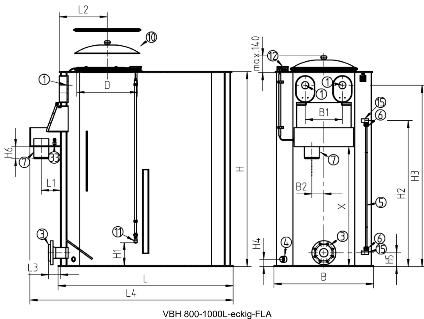
Fig. 1k: Maßbild Vorbehälter VBH 800-1000L-eckig-FLA
