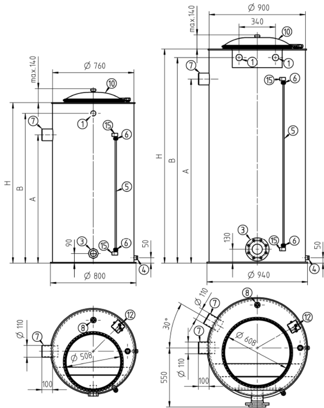
VBH 150-600L-rund-GII
