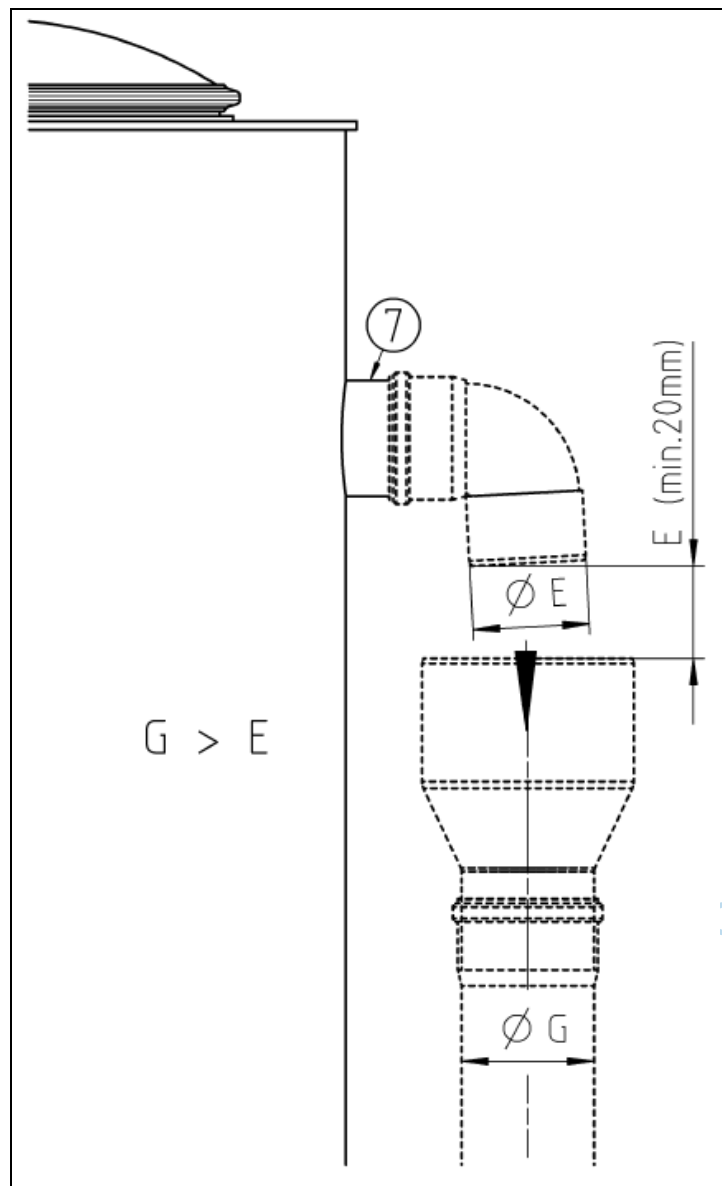
Fig. 6c: Demontage der Klappe am Überlauf FLA
