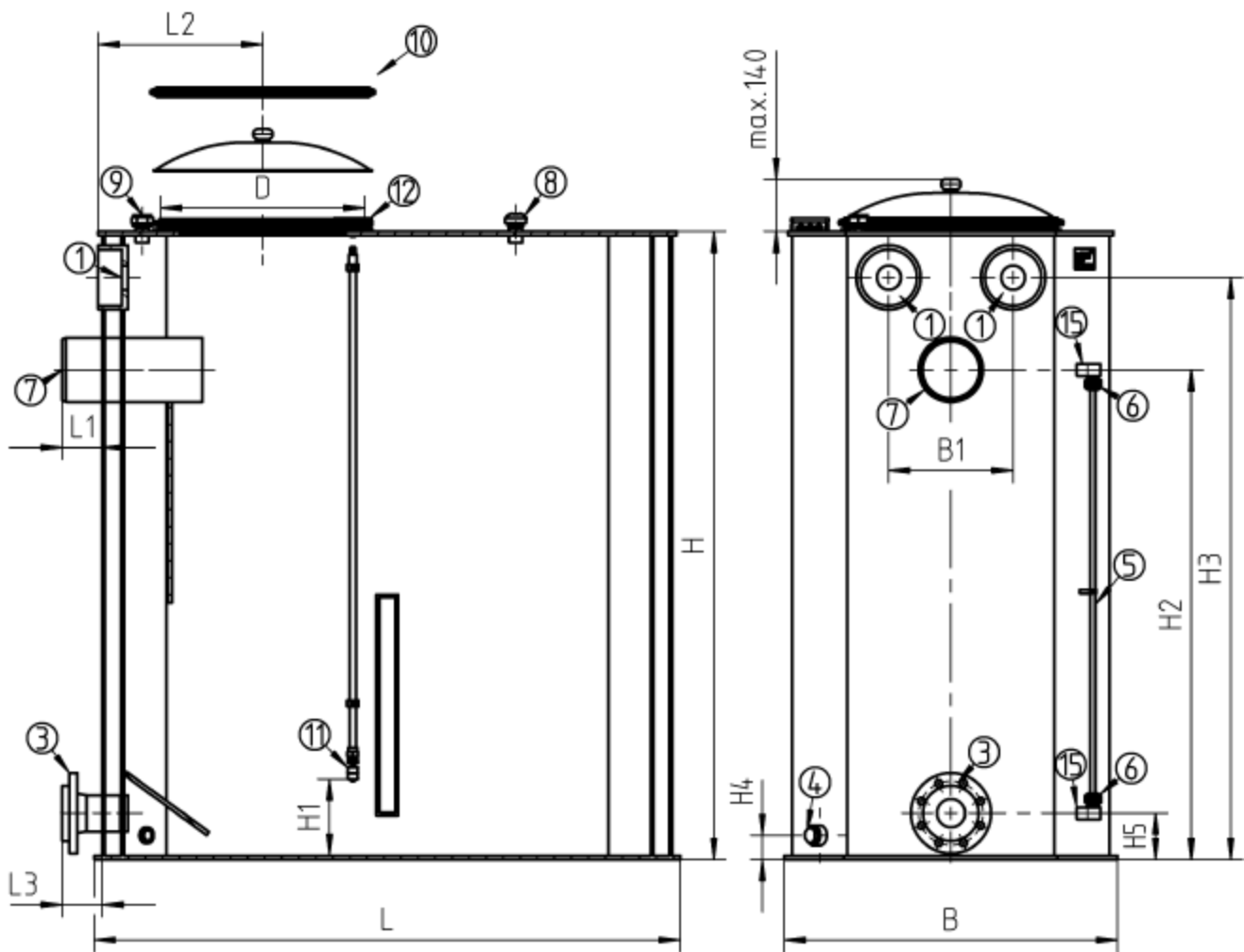
VBH 800-1000L-eckig-GIII
