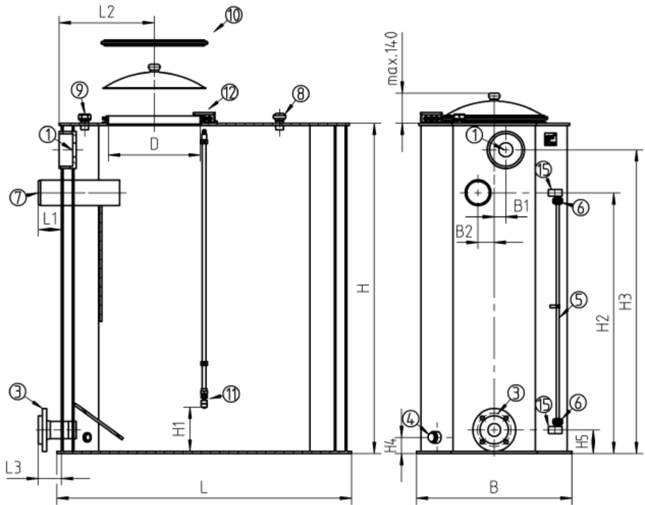
VBH 150-500L-eckig-GIII
