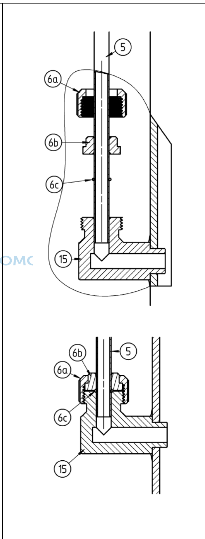
Fig. 2b: Verschraubung Wasserstandsanzeige
