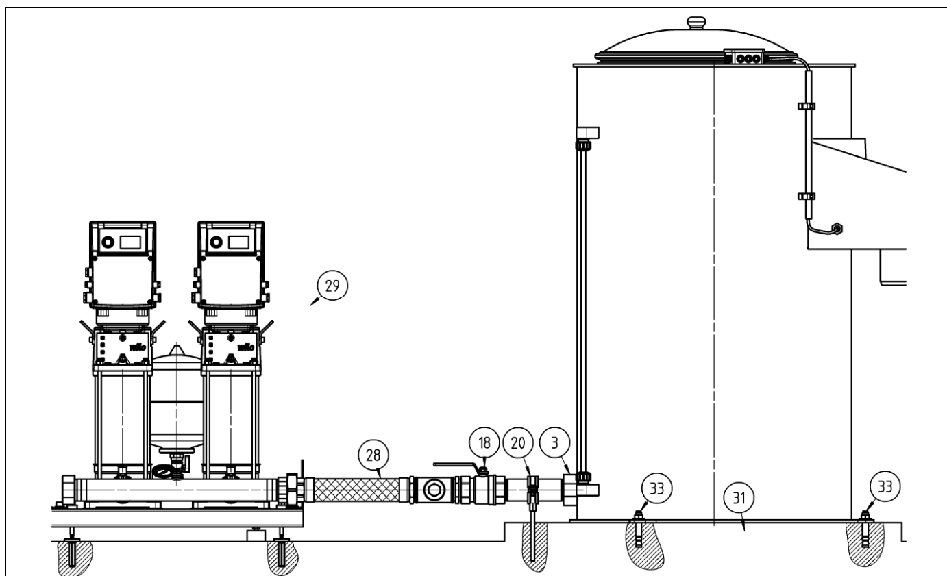
Fig. 5b: Beispiel Anschluss Druckerhöhungsanlage mit Flanschanschluss
