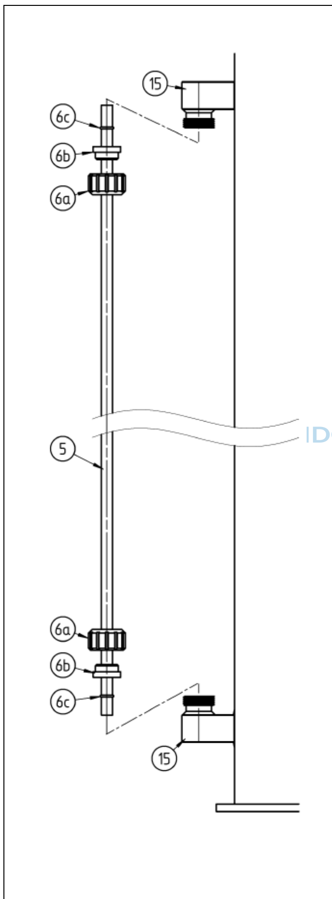
Fig. 2a: Wasserstandsanzeige
