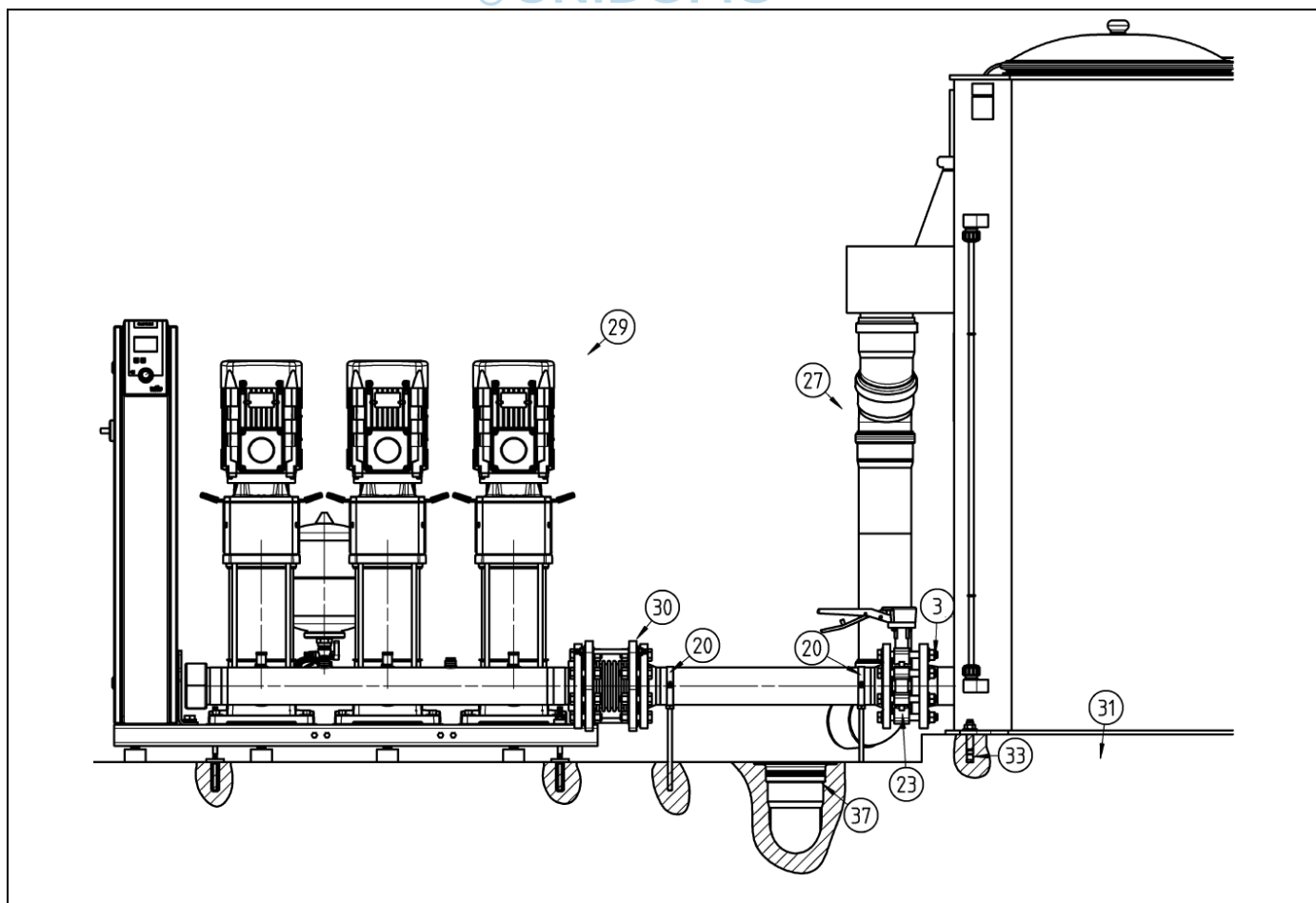
Fig. 5b: Beispiel Anschluss Druckerhöhungsanlage mit Flanschanschluss
