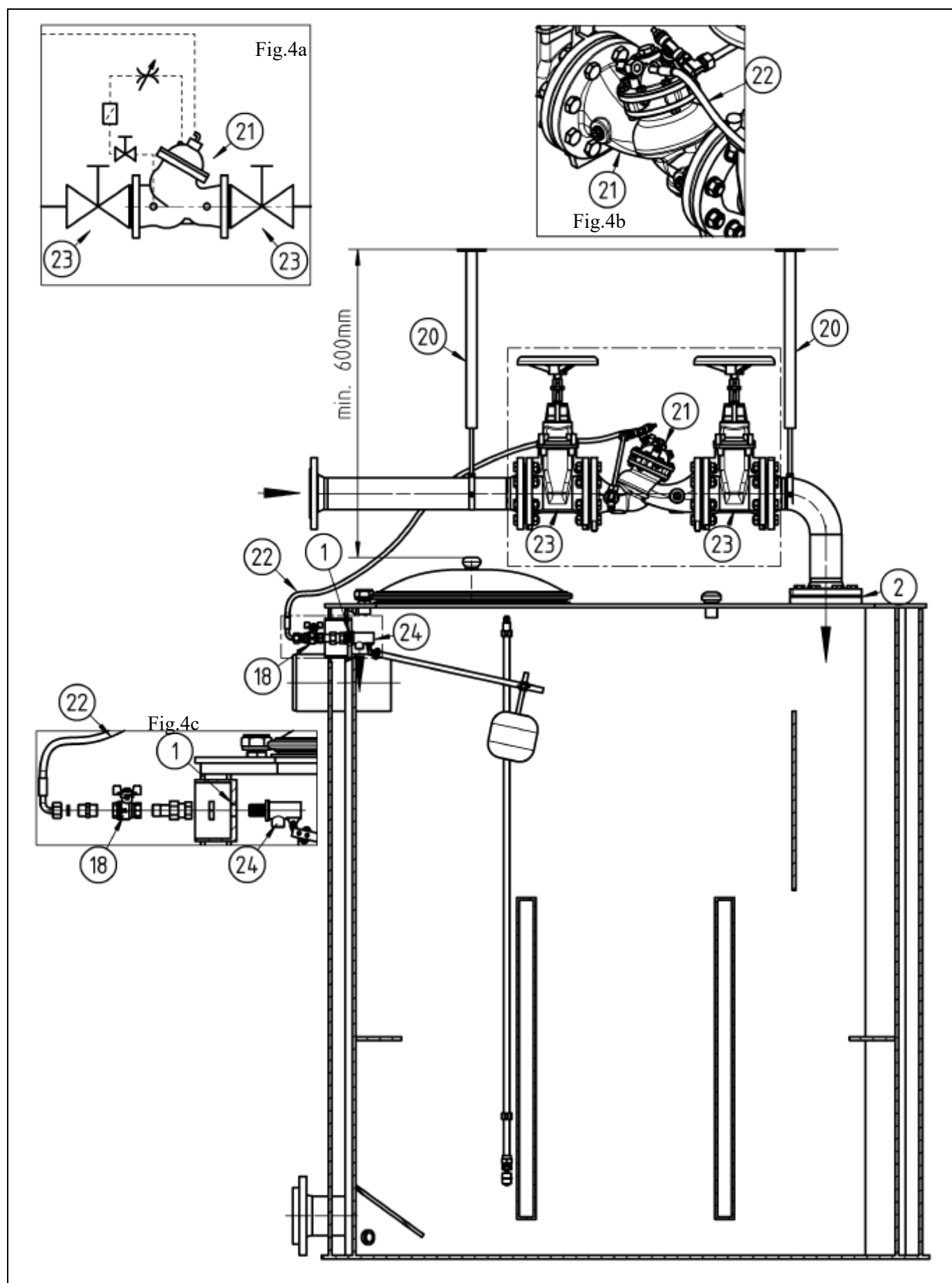
Fig. 4: Einbaubeispiel Membranventil
