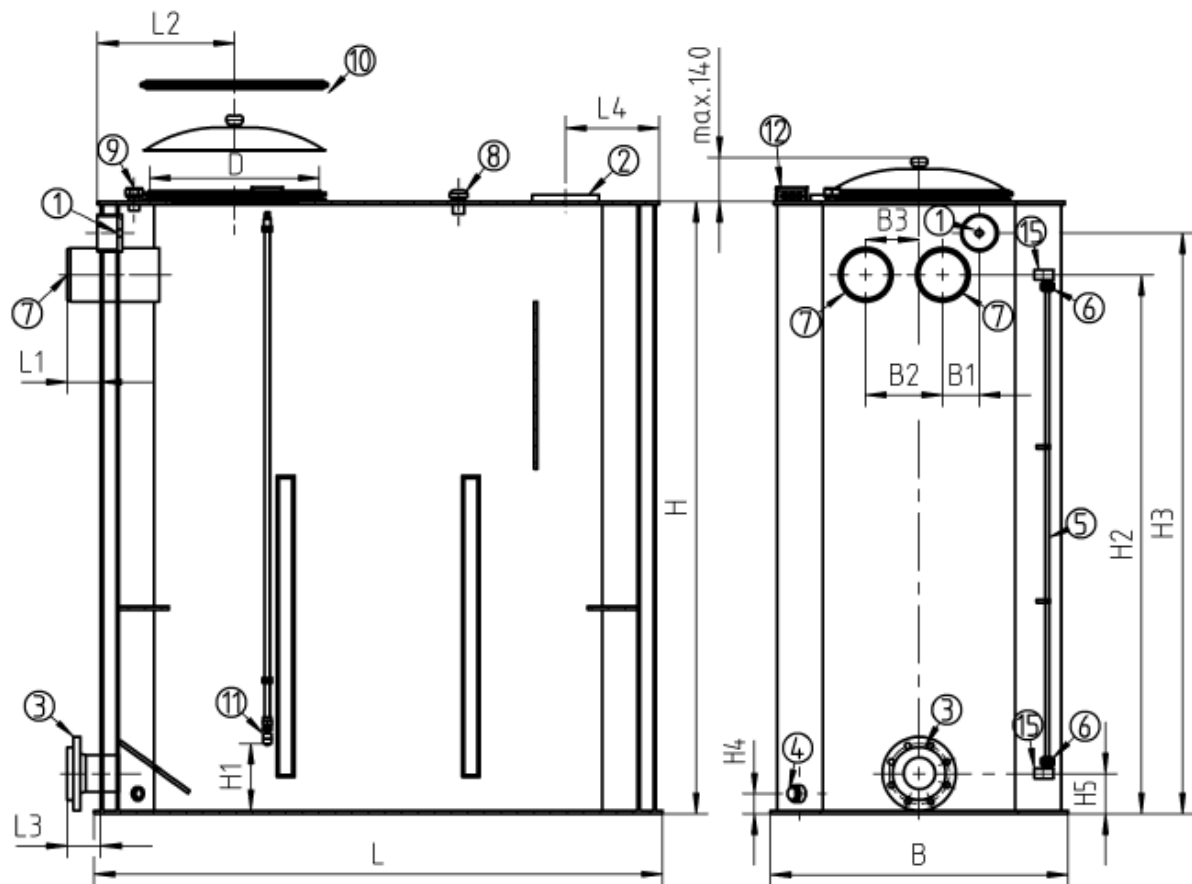
VBH 1500-3000L-eckig-GIII
