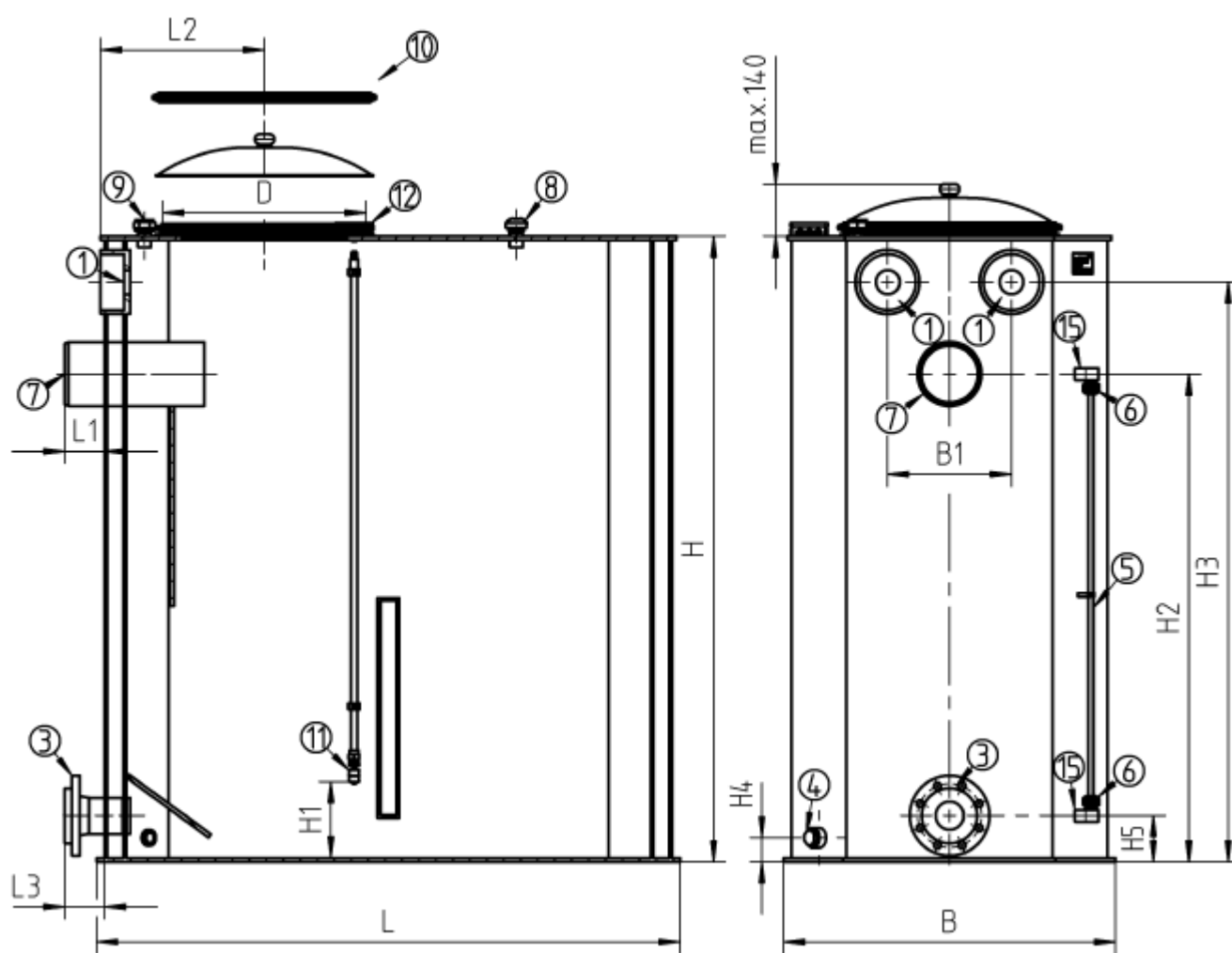
VBH 800-1000L-angular-GIII
