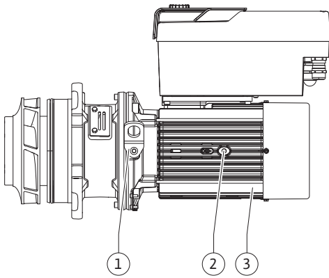
Fig. 4: Einstecksatz
