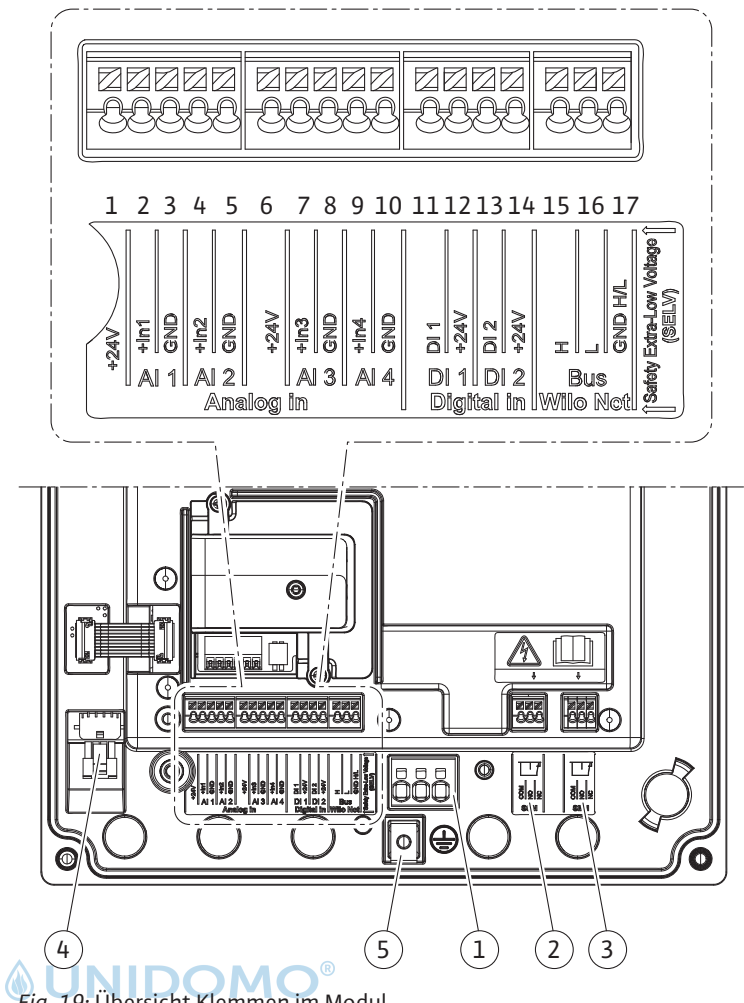
Fig. 19: Übersicht Klemmen im Modul
