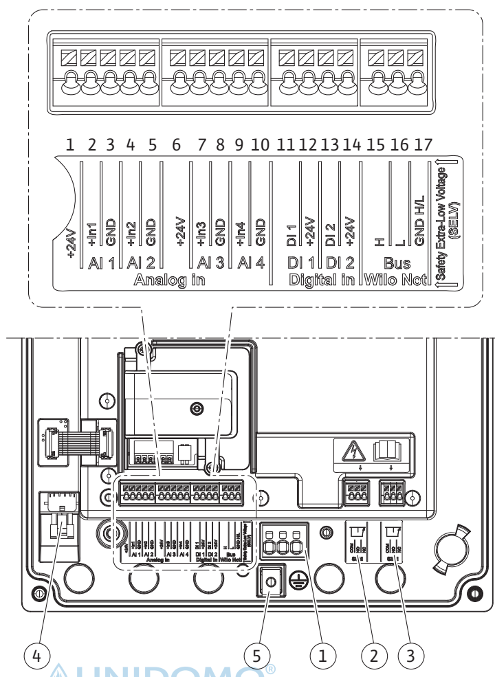
Fig. 19: Overzicht klemmen in de module
