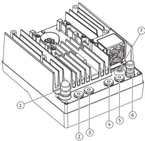
Fig. 18: Kabelverschraubungen/Kabelanschlüsse
