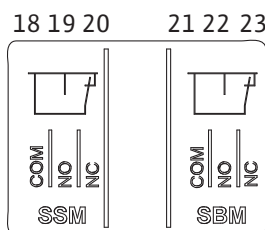
Fig. 23: Klemmen für SSM und SBM
