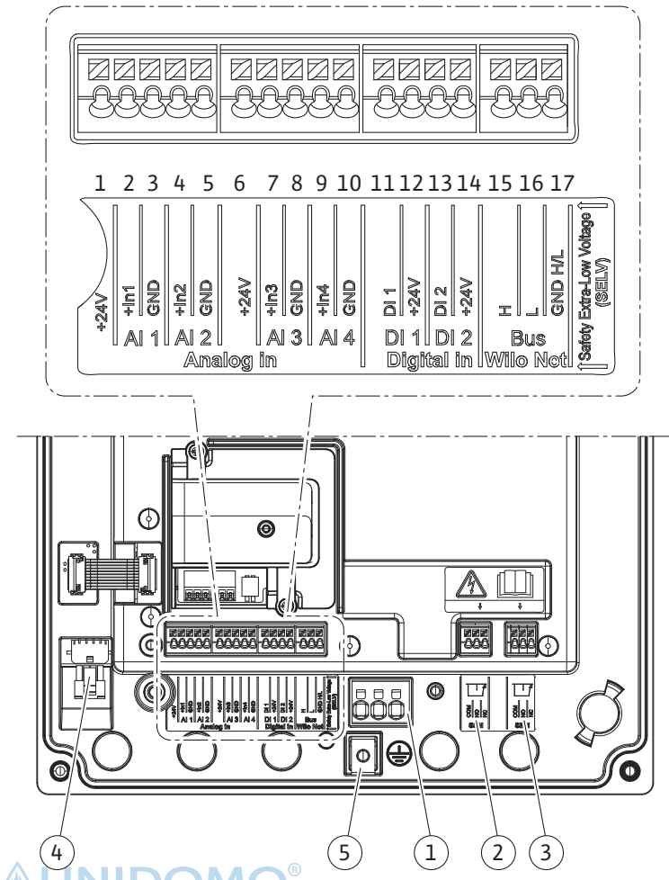
Fig. 19: Aperçu des bornes dans le module
