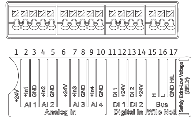
Fig. 20: Bornes pour les entrées analogiques, les entrées numériques et Wilo Net
