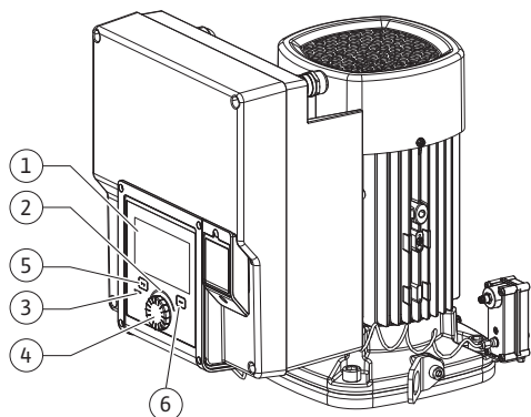
Fig. 28: Bedieningselementen
