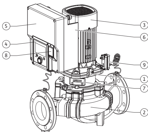
Fig. 1: Übersicht Pumpe
