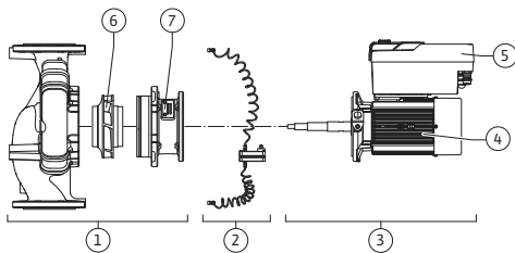
Fig. 3: Funktionsbaugruppen
