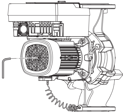
Fig. 5: Drehen der Welle
