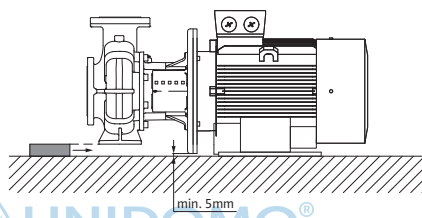
Corps de pompe soutenu, moteur fixé sur la fondation
