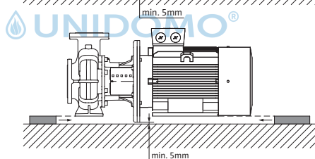
Corps de pompe et moteur soutenus
