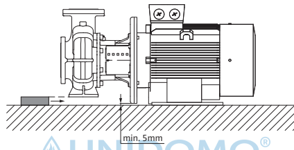
Pomphuis ondersteund, motor op fundament bevestigd
