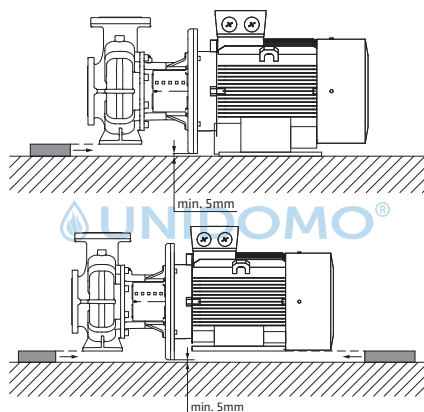
Pumpengehäuse unterstützt, Motor auf Fundament befestigt
