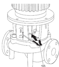
Fig. 13: Aanbrengen van de montagevork
