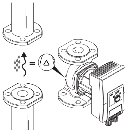
Fig. 6: Durchflussrichtung beachten
