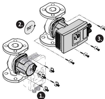
Fig. 15: Motor ausrichten
