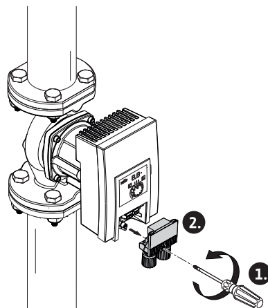
Fig. 19: Stecker demontieren®
