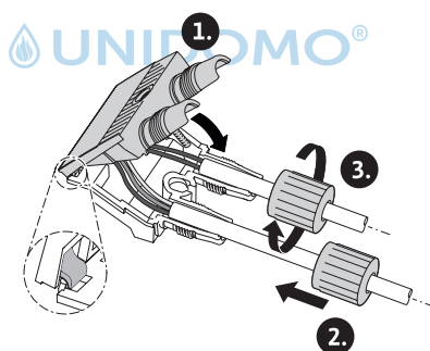
Fig. 23: Chiudere la spina
