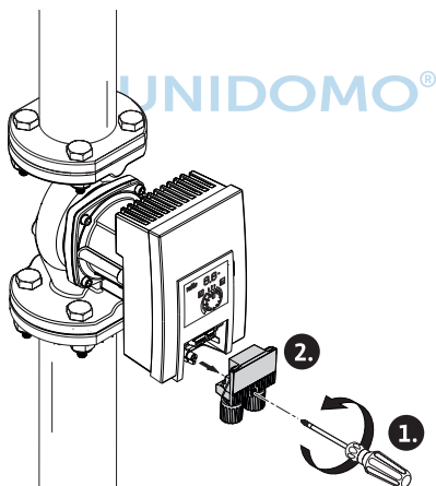
Fig. 19: Smontare la spina
