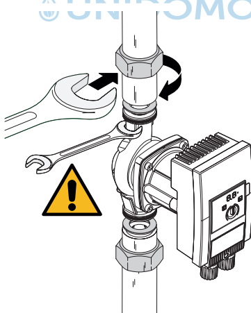
Fig. 9: Pumpe montieren
