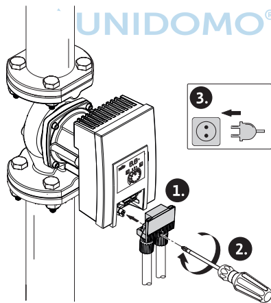
Fig. 24: Stecker montieren
