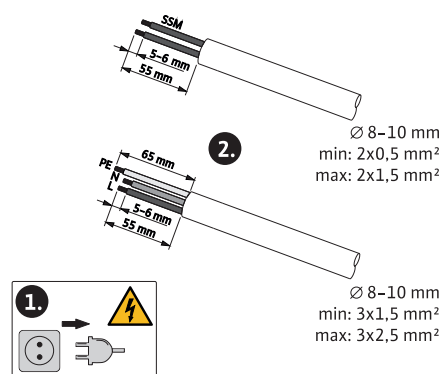
Fig. 18: Anschluss vorbereiten
