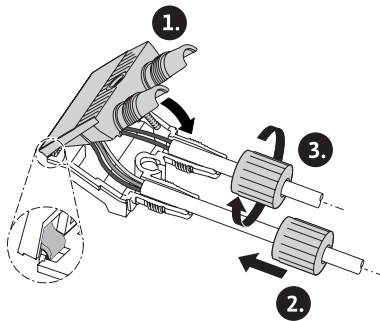
Fig. 23: Stecker schließen
