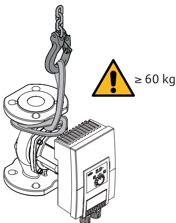
Fig. 5: Transportieren
