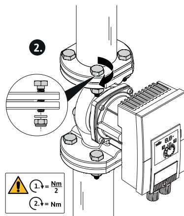
Fig. 13: Pumpe montieren
