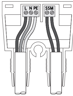
Fig. 22: Anschließen
