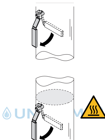
Fig. 14: Absperrarmaturen öffnen
