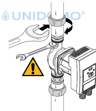
Fig. 9: Montare la pompa
