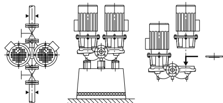
Fig. 9: Aanzicht DL
