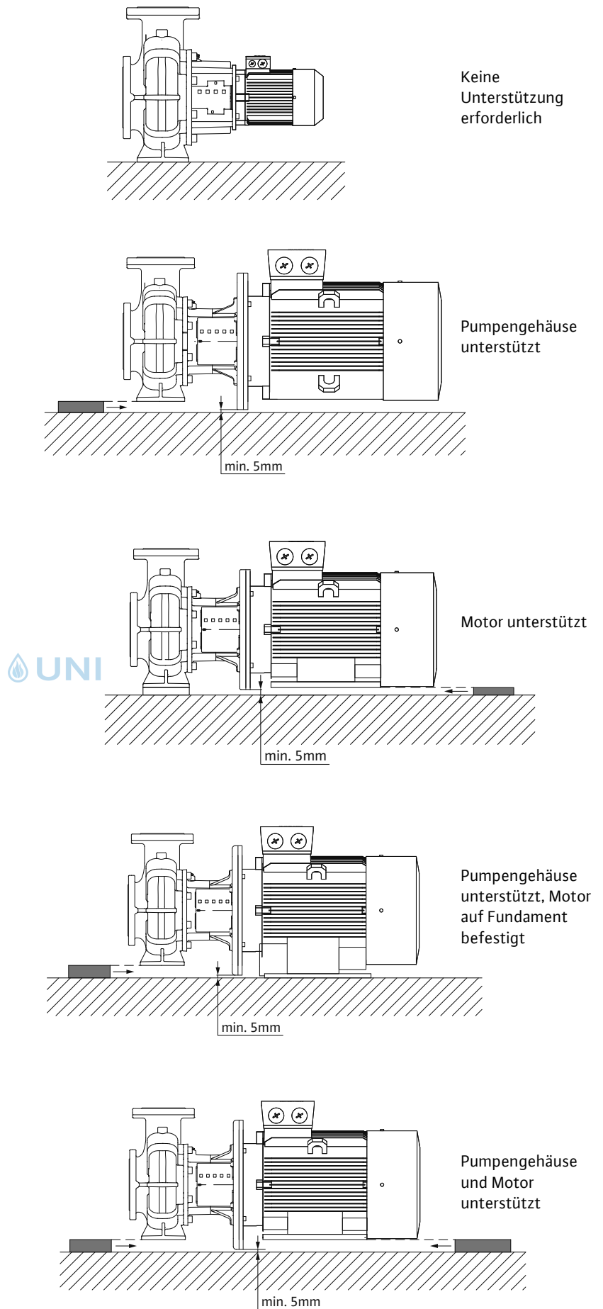
Fig. 14: Einbaubeispiele BL
