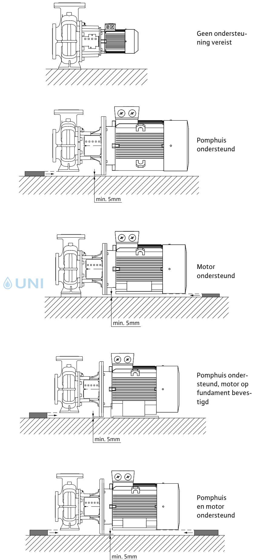
Fig. 14: Installatievoorbeeld BL
