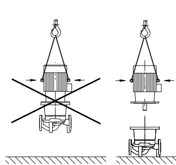
Fig. 7: Transport des Motors
