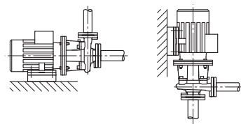
Fig. 41: Version BL
