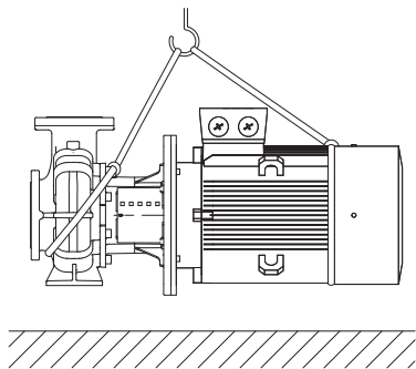
Fig. 33: Positionnement des élingues de charge (version BL)
