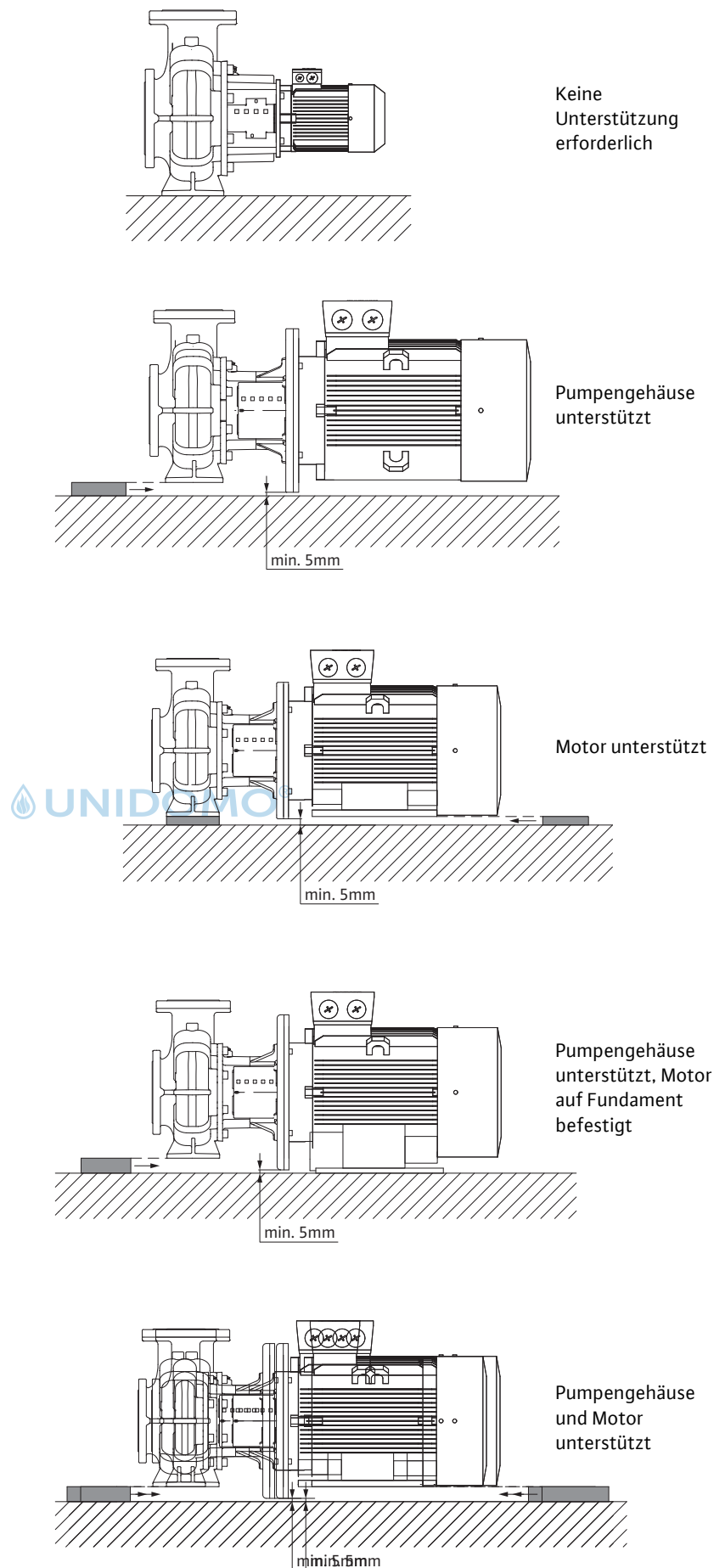
Fig. 42: Einbaubeispiele BL
