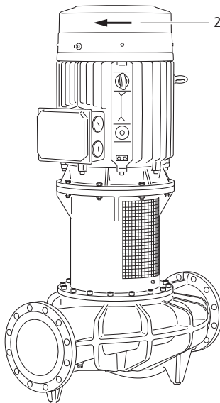
Fig. 47: Drehrichtung überprüfen
