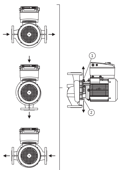
Afb. 18: Toegestane inbouwposities met horizontale motoras
