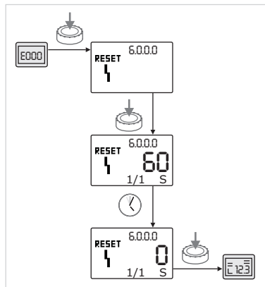
Afb. 45: Fouttype A of D bevestigen
