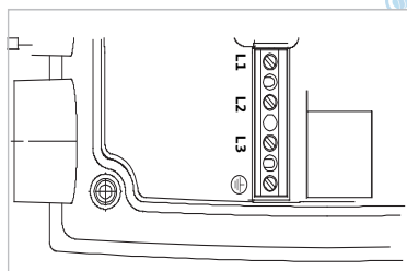
Fig. 24: Leistungsklemmen (Netzanschlussklemmen)
