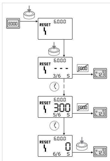
Fig. 50: Fehlertyp C quittieren
