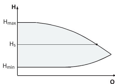
Afb. 10: Regeling \Delta p-c
