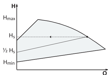
Afb. 11: Regeling \Delta p-v
