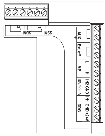
Afb. 23: Stuurklemmen
