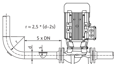
Fig. 21: Section de stabilisation en amont et en aval de la pompe
