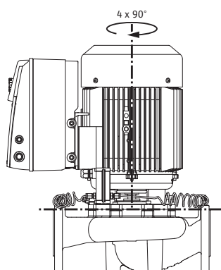
Afb. 19: Toegestane inbouwposities met verticale motoras
