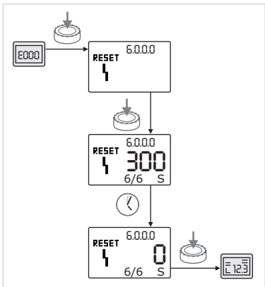
Afb. 48: Fouttype B bevestigen (X = Y)
