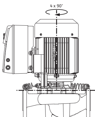
Fig. 19: Zulässige Einbaulagen mit vertikaler Motorwelle
