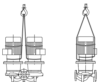
Fig. 7: Transport der Pumpe
