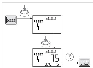
Afb. 47: Fouttype B bevestigen (X &lt; Y)
