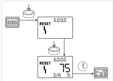
Fig. 47: Acquittement du type de défaut B (X < Y)
