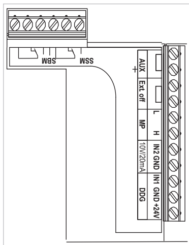
Fig. 23: Steuerklemmen
