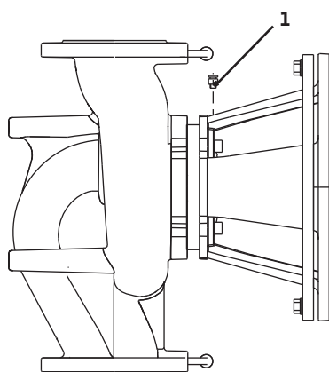
Fig. 38: Entlüftungsventil
