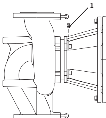
Fig. 38: Soupape d'échappement
