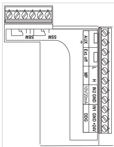
Fig. 23: Bornes de commande
