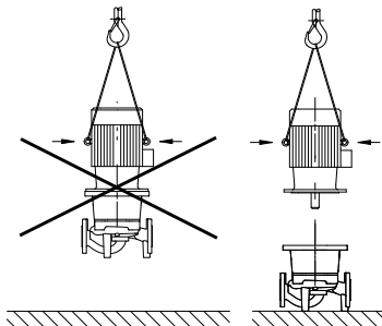
Afb. 8: Transport van de motor
