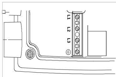
Afb. 24: Vermogensklemmen (netaansluitklemmen)
