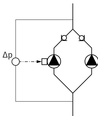
Afb. 13: Voorbeeld, aansluiting verscheldruksensor
