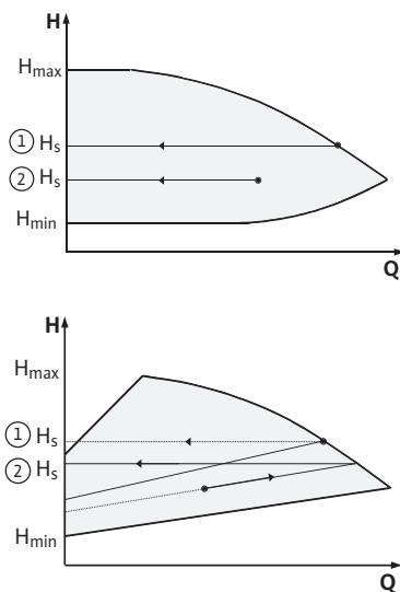
Fig. 40: Regelung \Delta p -c/ \Delta p -v
