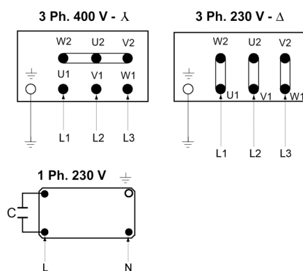
Fig. 3: alimentación eléctrica
