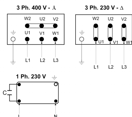
Fig. 3: Netzanschluss
