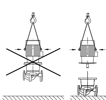
Fig. 6: Transport des Motors (Prinzipdarstellung)
