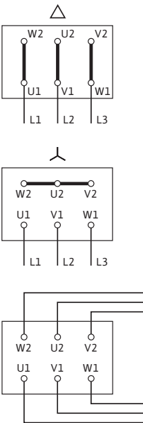
Fig. 11: Alimentation réseau
