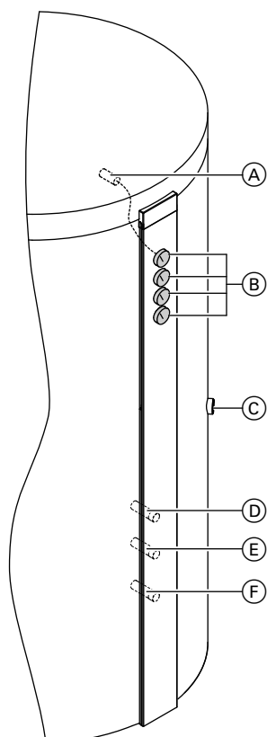
Abb. 4 Vorderseite, Ansicht ohne angebaute Solar-Divicon (Zubehör)
