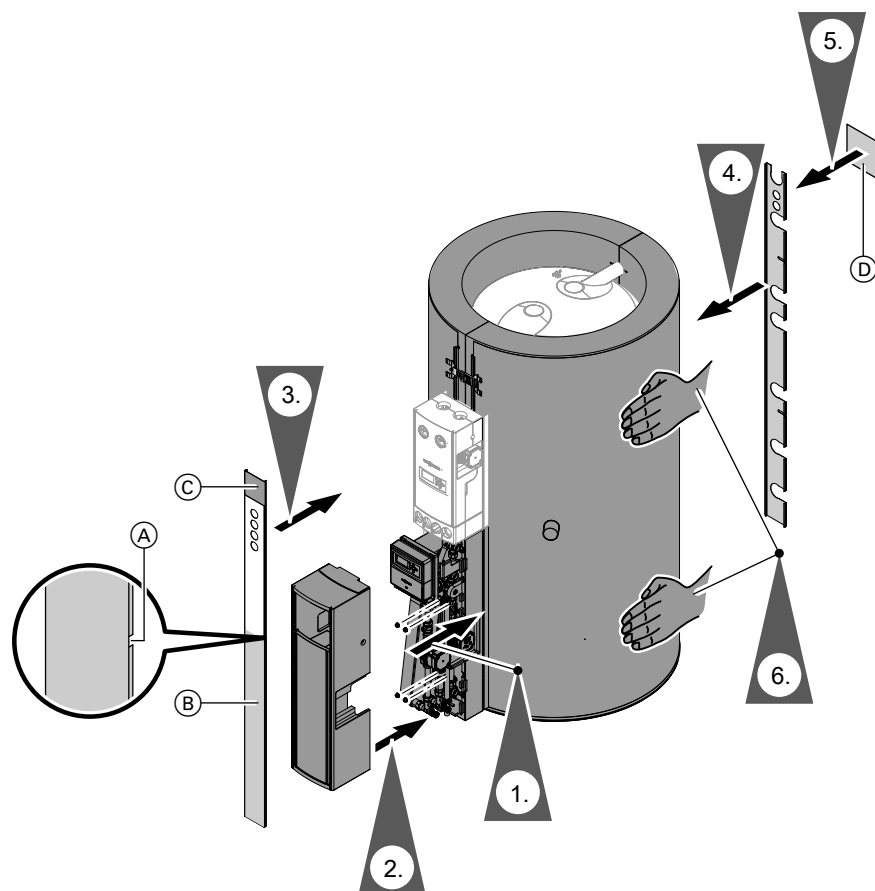
Abb. 32 Beispiel: Vitocell 140-E, Typ SEIC, 750 l
