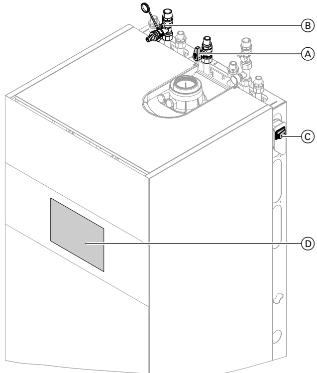
Abb. 16 Beispiel mit Anschlüssen nach oben
