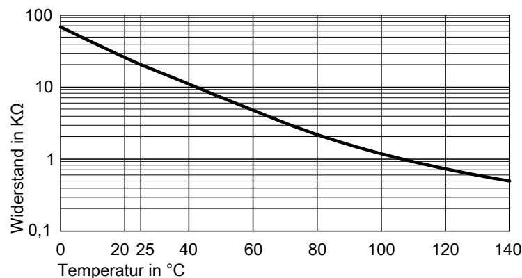
Abb. 50 Sensortyp: NTC 20 kΩ
