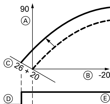
Abb. 55 Beispiel 1: Änderung des Raumtemperatur-Sollwerts von 20 auf 26 °C
