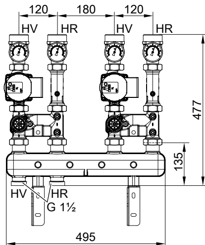
Abb. 4 Darstellung ohne Wärmedämmung, ohne Mischer-Motor und ohne Erweiterungssatz Mischer
