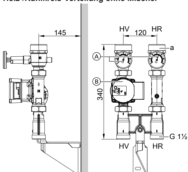
Abb. 3 Heiz-/Kühlkreis-Verteilung ohne Mischer: Wandmontage, Darstellung ohne Wärmedämmung
