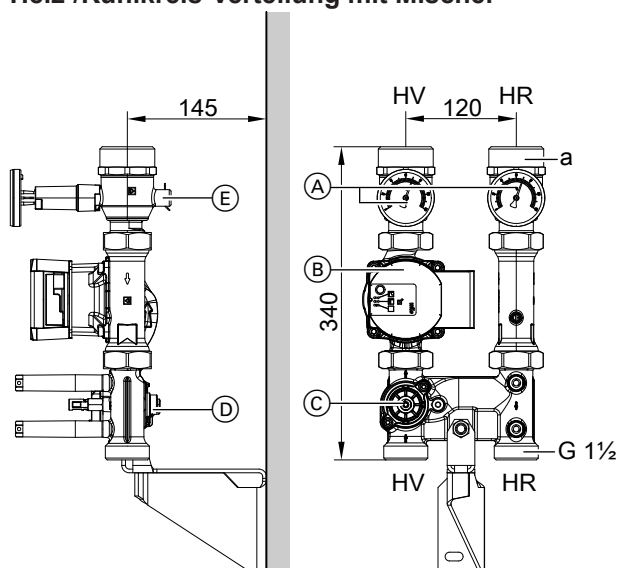
Abb. 2 Heiz-/Kühlkreis-Verteilung mit Mischer: Wandmontage, Darstellung ohne Wärmedämmung, ohne Mischer-Motor und ohne Erweiterungssatz Mischer
