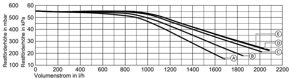
Abb. 67 Mit Umwälzpumpe Grundfos UPM3S 25-60, Typen M3-20-KM-G-A, M3-20-PL-G-A, M3-20-XX-G-A
