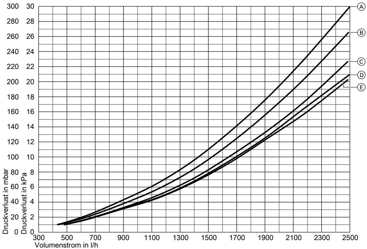
Abb. 65 Mit Umwälzpumpe Grundfos UPM3K 25-70, Typen M3-32-KM-G-A, M3-32-PL-G-A, M3-32-XX-G-A
