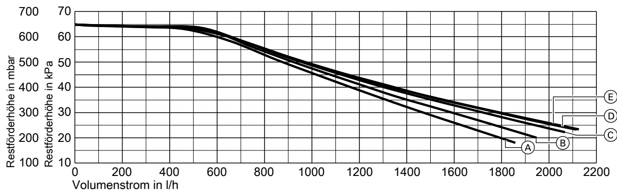
Abb. 68 Mit Umwälzpumpe Wilo PARA 25/6, Typen M3-25-KM-W-A, M3-25-PL-W-A, M3-25-XX-W-A
