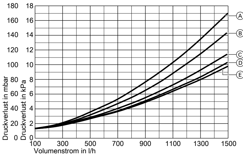
Abb. 63 Mit Umwälzpumpe Grundfos UPM3S 25-60, Typen M3-25-KM-G-A, M3-25-PL-G-A, M3-25-XX-G-A
