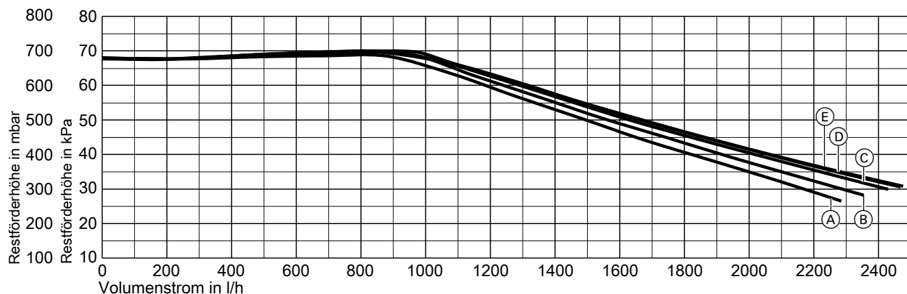
Abb. 71 Mit Umwälzpumpe Grundfos UPM3K 25-70, Typen M3-32-KM-G-A, M3-32-PL-G-A, M3-32-XX-G-A
