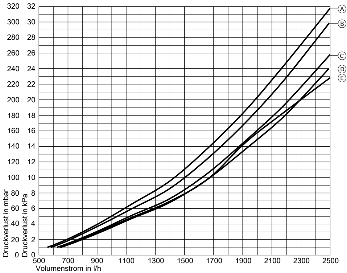
Abb. 64 Mit Umwälzpumpe Wilo PARA 25/8, Typen M3-32-KM-W-A, M3-32-PL-W-A, M3-32-XX-W-A
