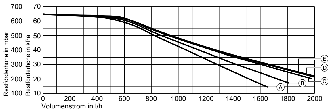
Abb. 66 Mit Umwälzpumpe Wilo PARA 25/6, Typen M3-20-KM-W-A, M3-20-PL-W-A, M3-20-XX-W-A
