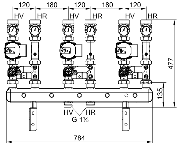
Abb. 5 Darstellung ohne Wärmedämmung, ohne Mischer-Motor und ohne Erweiterungssatz Mischer
