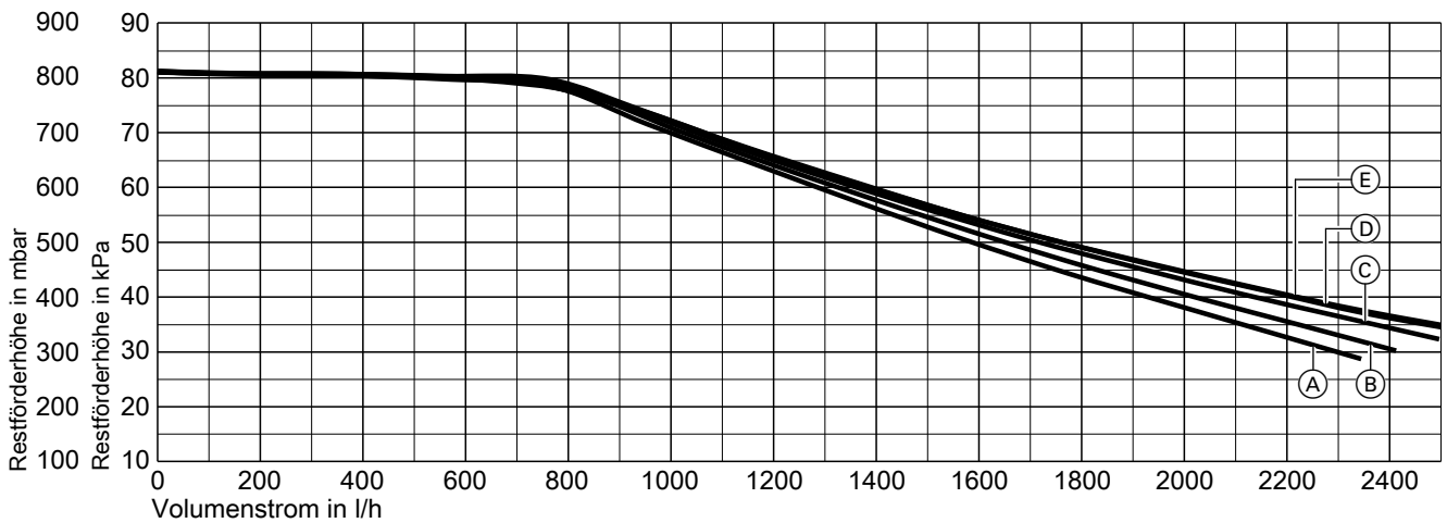
Abb. 70 Mit Umwälzpumpe Wilo PARA 25/8, Typen M3-32-KM-W-A, M3-32-PL-W-A, M3-32-XX-W-A
