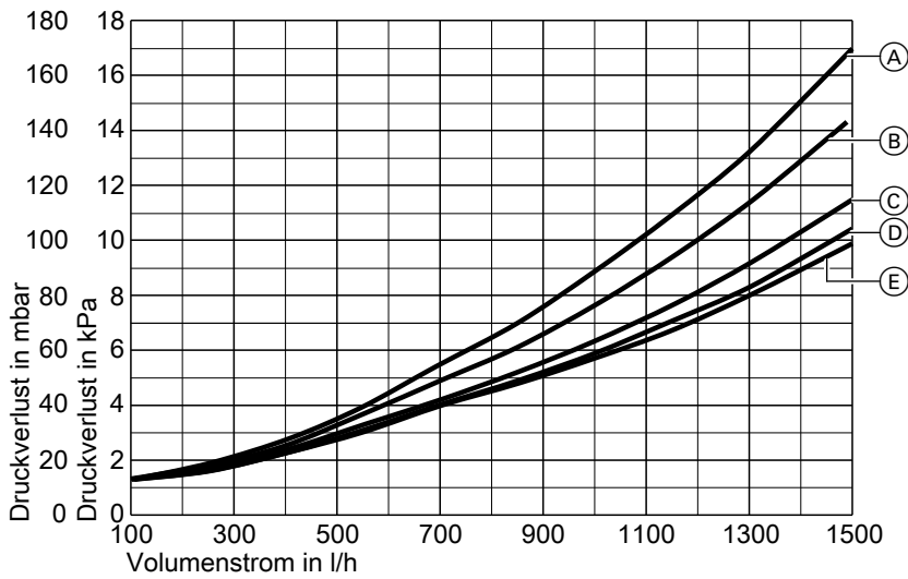
Abb. 62 Mit Umwälzpumpe Wilo PARA 25/6, Typen M3-25-KM-W-A, M3-25-PL-W-A, M3-25-XX-W-A
