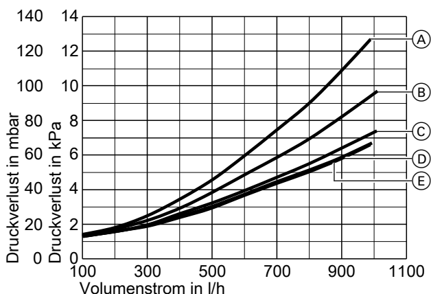
Abb. 60 Mit Umwälzpumpe Wilo PARA 25/6, Typen M3-20-KM-W-A, M3-20-PL-W-A, M3-20-XX-W-A
