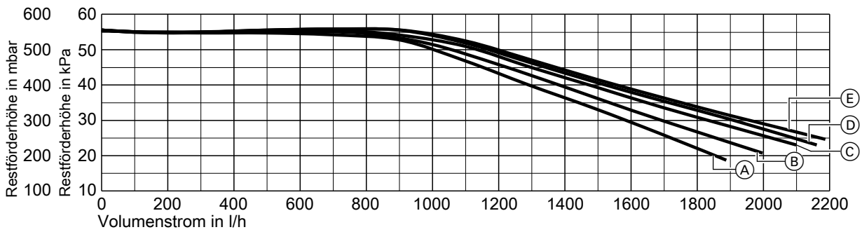
Abb. 69 Mit Umwälzpumpe Grundfos UPM3S 25-60, Typen M3-25-KM-G-A, M3-25-PL-G-A, M3-25-XX-G-A
